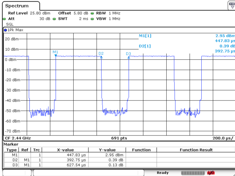
Bluetooth - LE1Mbps
