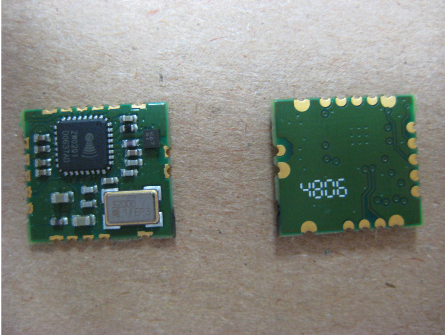
RF Module Assembly
