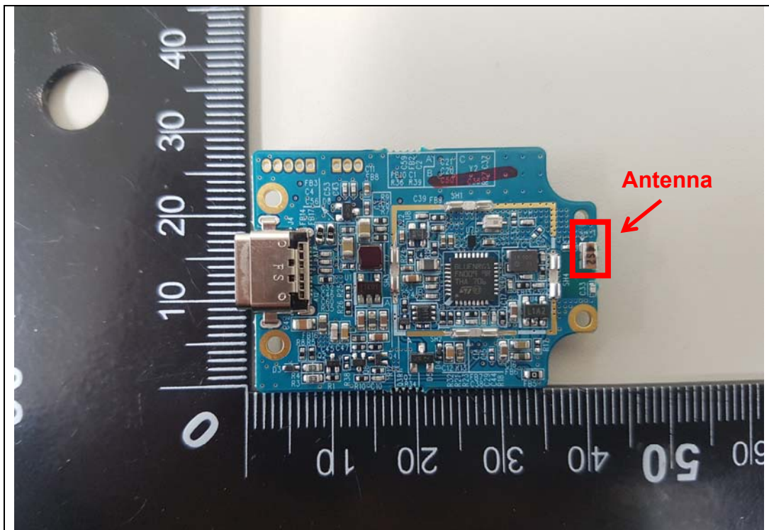
Antenna (2.4 GHz)
