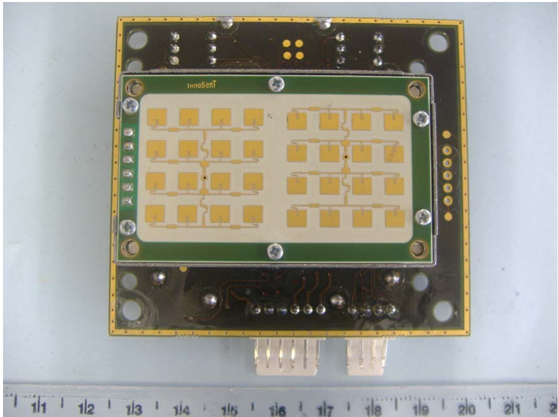
Assemble EUT RF Module Side
