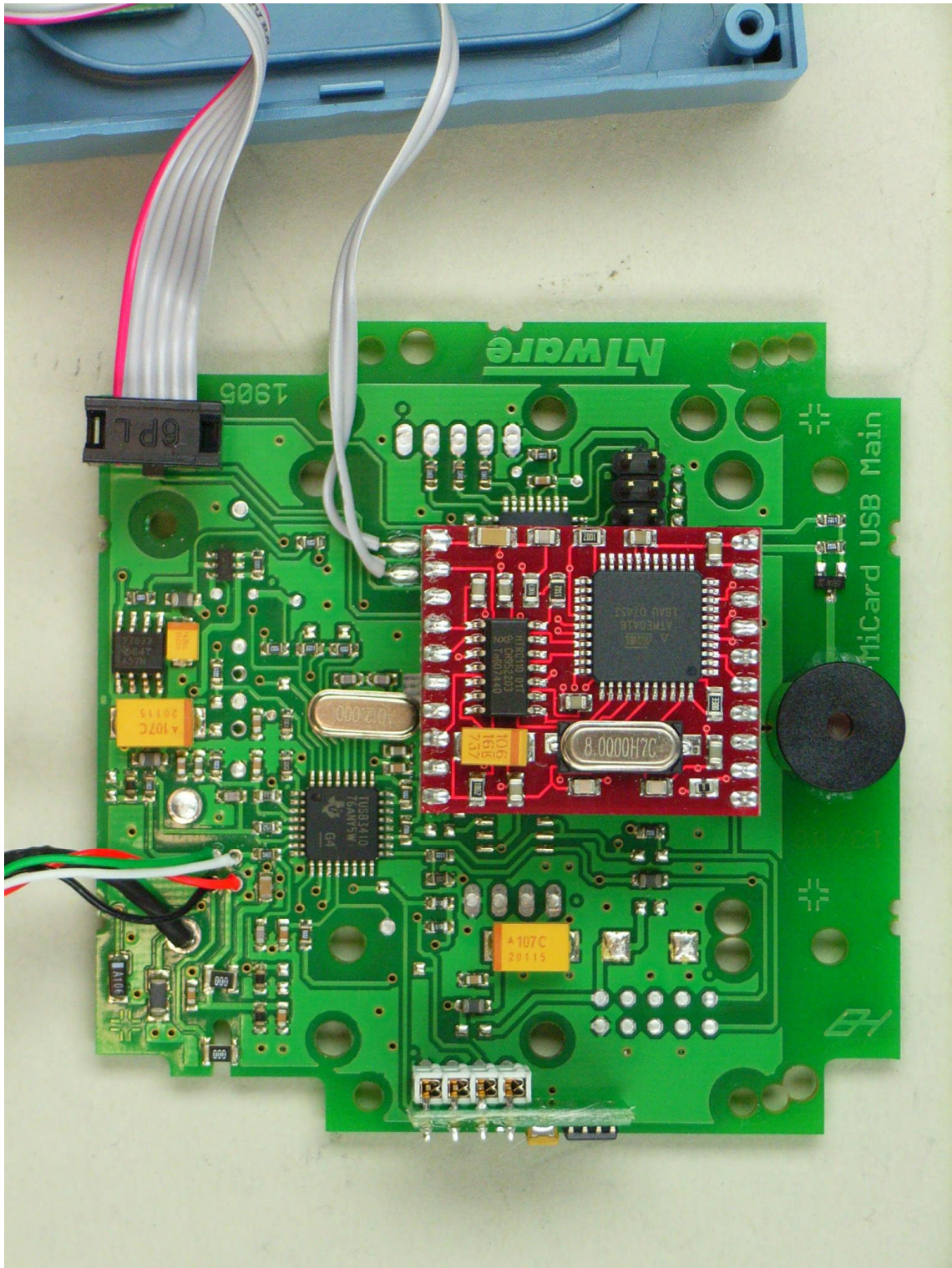
81609eut7: EUT, main-PCB, top view
