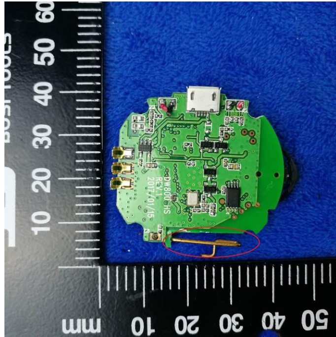
Antenna View(PP)
