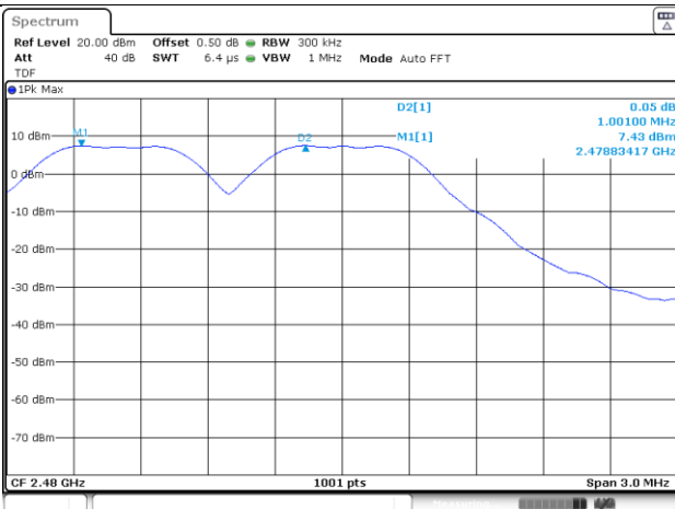
2 480 MHz
