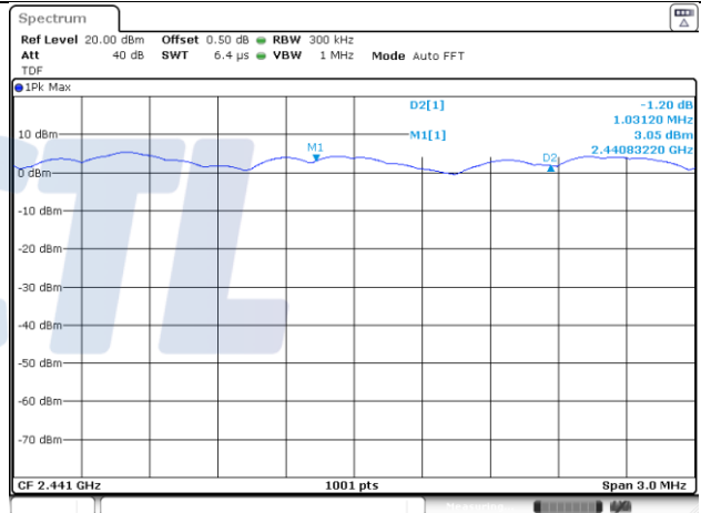
2 441 MHz
