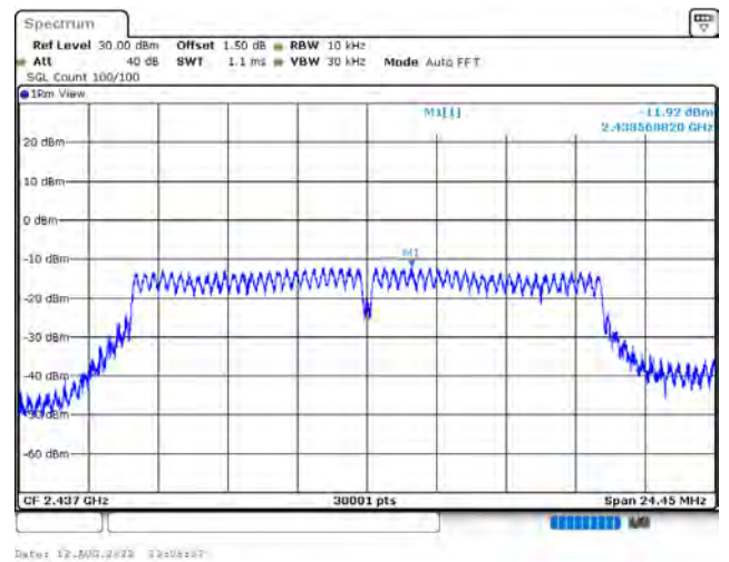
802.11g / 2437 MHz
