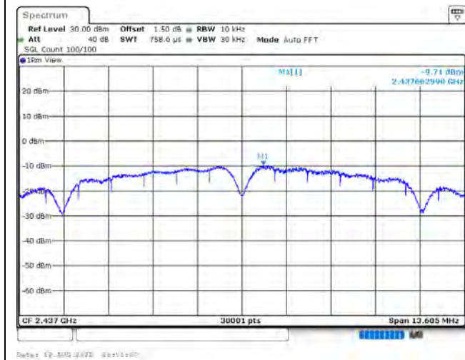
802.11b / 2437 MHz
