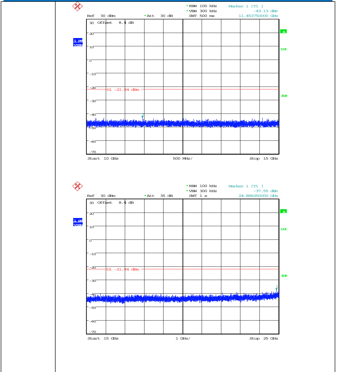
\pi/4 DQPSK MCH_Graphs
