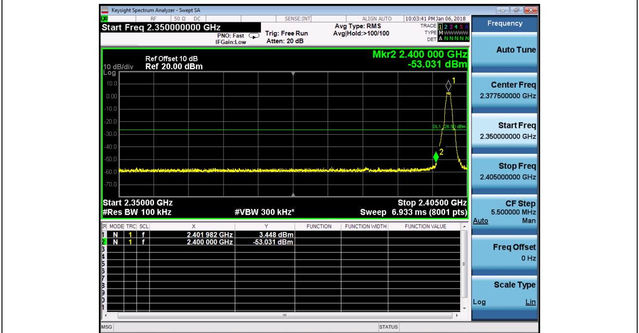
Mode 1 CH00 (2402MHz)
