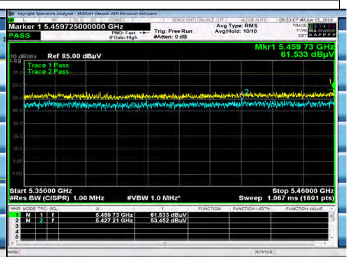
802.11ac-VHT 5290M(5350-5460MHz)
