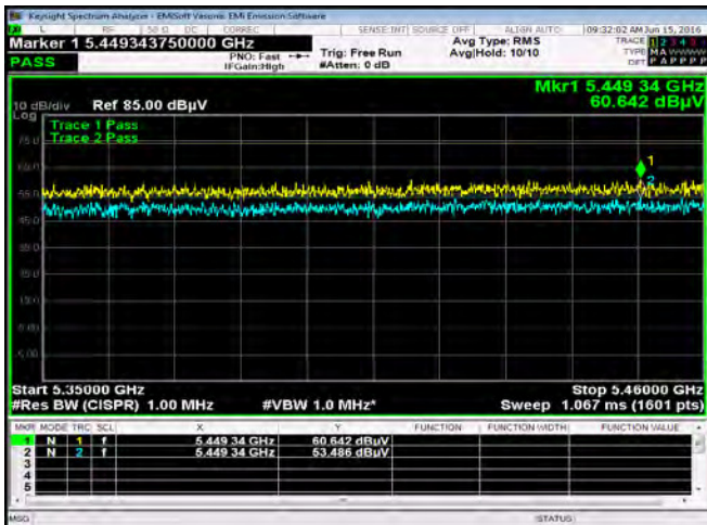
802.11a 5500M(5350-5460MHz)
