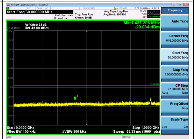
30MHz-1000MHz
