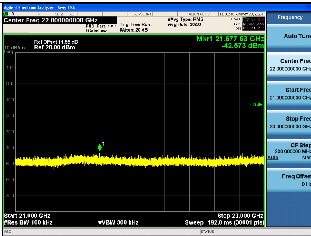
BLE_500K-Ant1-2440-21000~23000-PASS
