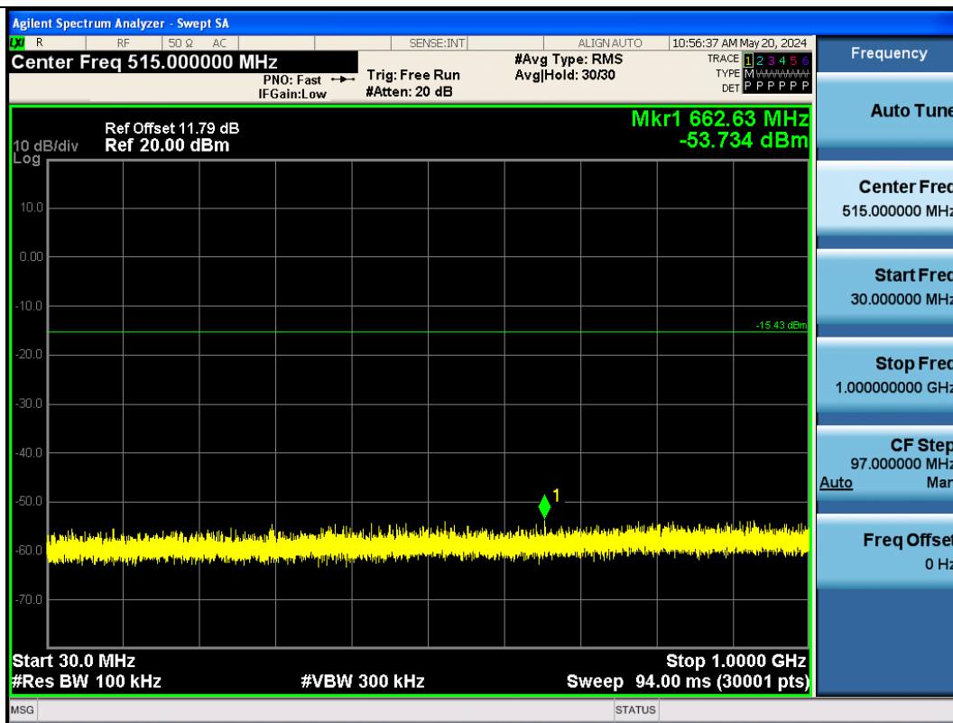
BLE_500K-Ant1-2402-30~1000-PASS
