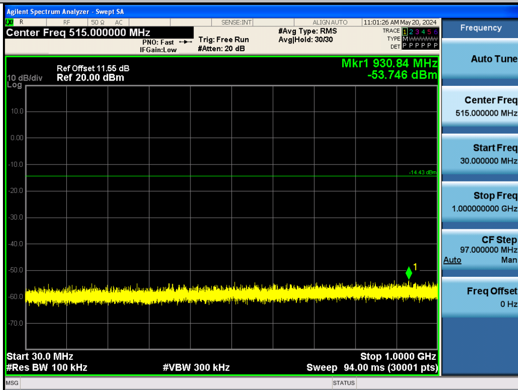
BLE_500K-Ant1-2440-30~1000-PASS
