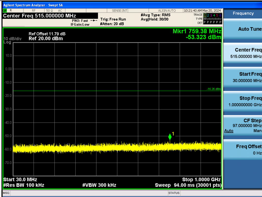
BLE_2M-Ant1-2402-30~1000-PASS
