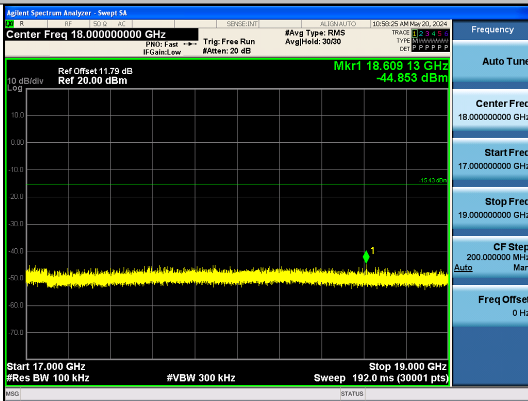
BLE_500K-Ant1-2402-17000~19000-PASS
