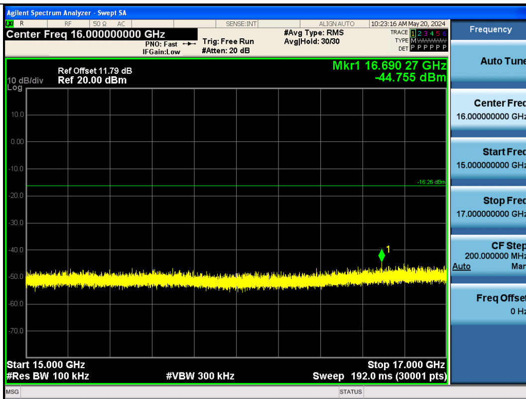
BLE_2M-Ant1-2402-15000~17000-PASS
