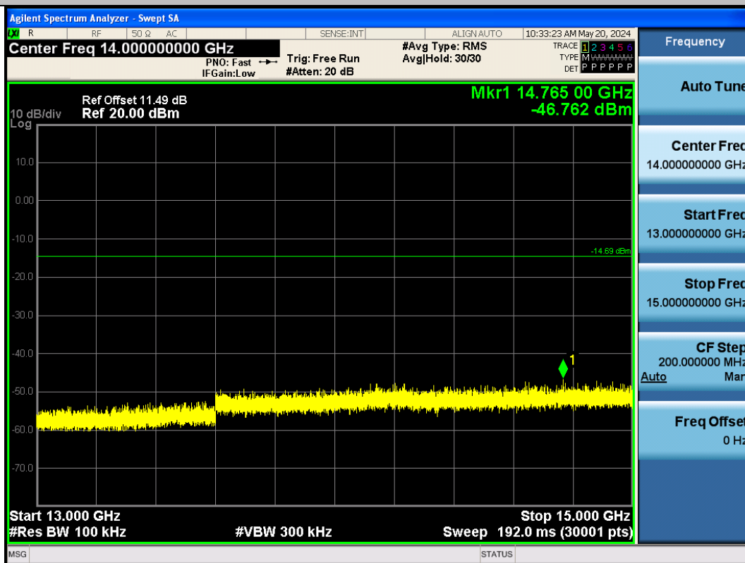
BLE_2M-Ant1-2480-13000~15000-PASS
