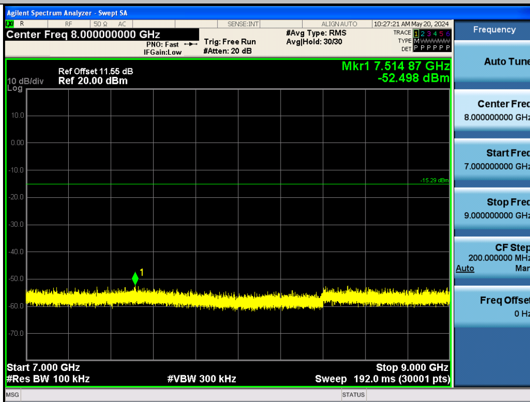
BLE_2M-Ant1-2440-7000~9000-PASS
