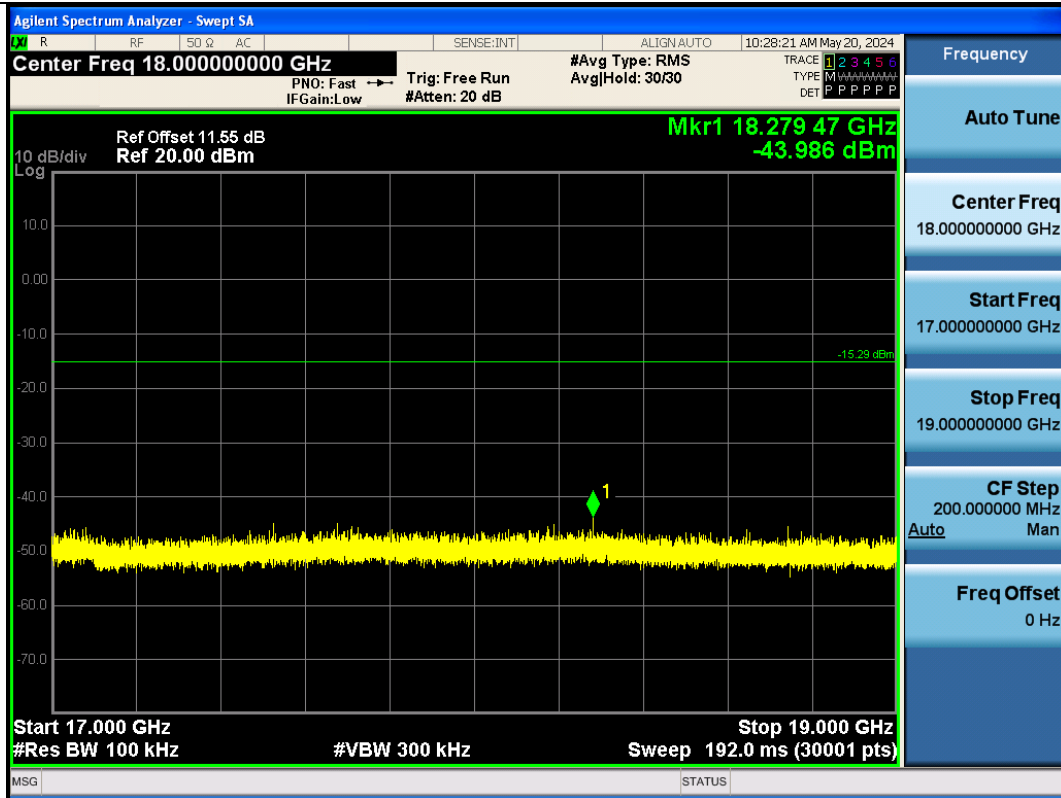
BLE_2M-Ant1-2440-17000~19000-PASS
