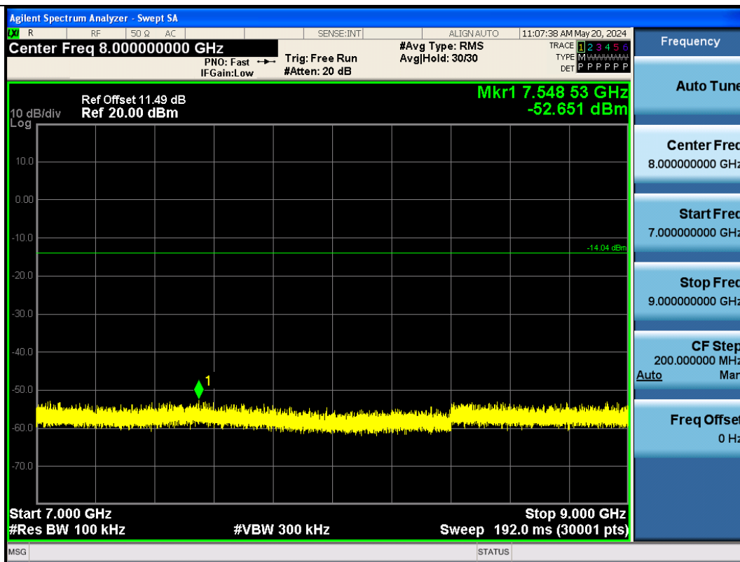
BLE_500K-Ant1-2480-7000~9000-PASS
