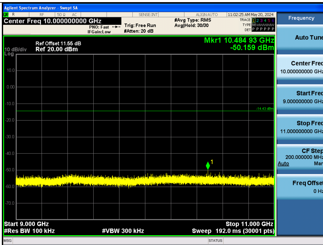
BLE_500K-Ant1-2440-9000~11000-PASS
