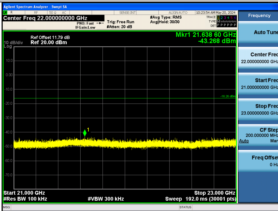
BLE_2M-Ant1-2402-21000~23000-PASS
