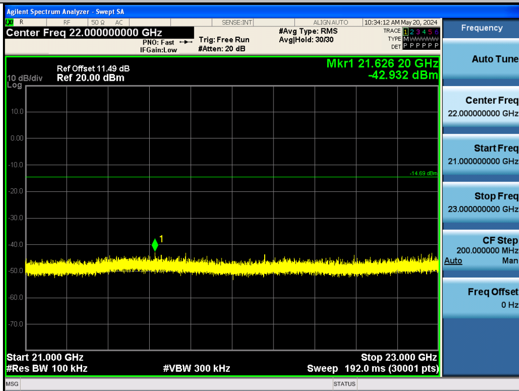
BLE_2M-Ant1-2480-21000~23000-PASS
