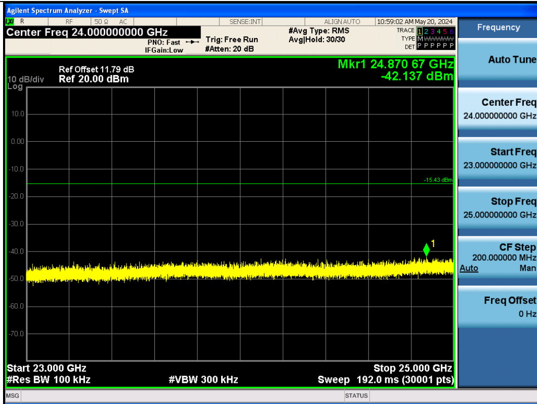
BLE_500K-Ant1-2402-23000~25000-PASS
