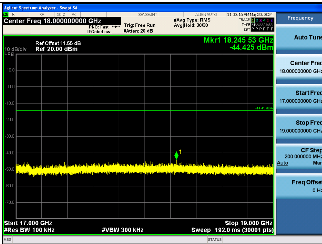
BLE_500K-Ant1-2440-17000~19000-PASS
