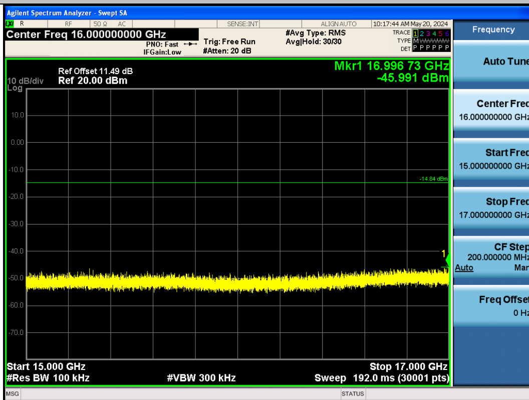
BLE_1M-Ant1-2480-15000~17000-PASS
