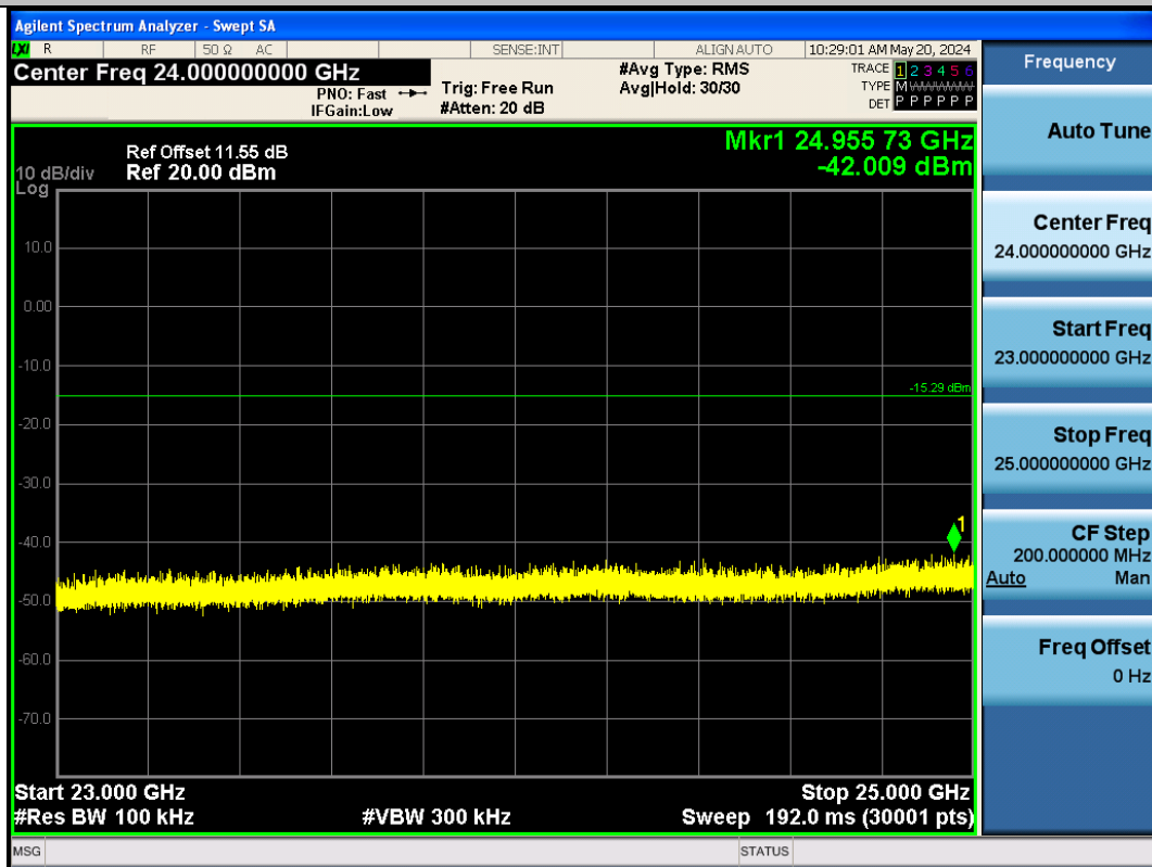
BLE_2M-Ant1-2440-23000~25000-PASS
