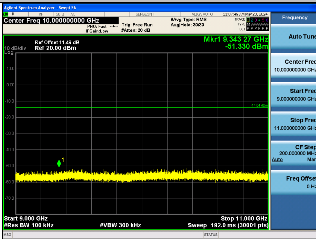
BLE_500K-Ant1-2480-9000~11000-PASS
