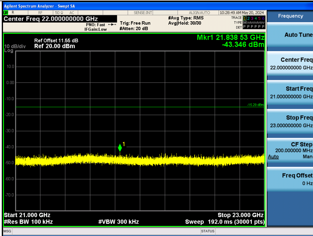
BLE_2M-Ant1-2440-21000~23000-PASS
