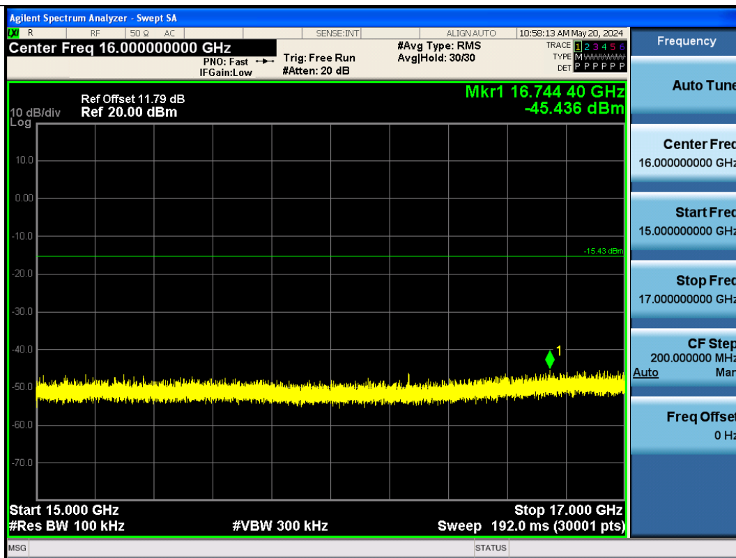
BLE_500K-Ant1-2402-15000~17000-PASS
