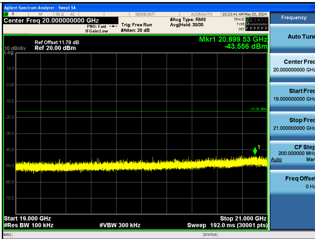
BLE_2M-Ant1-2402-19000~21000-PASS
