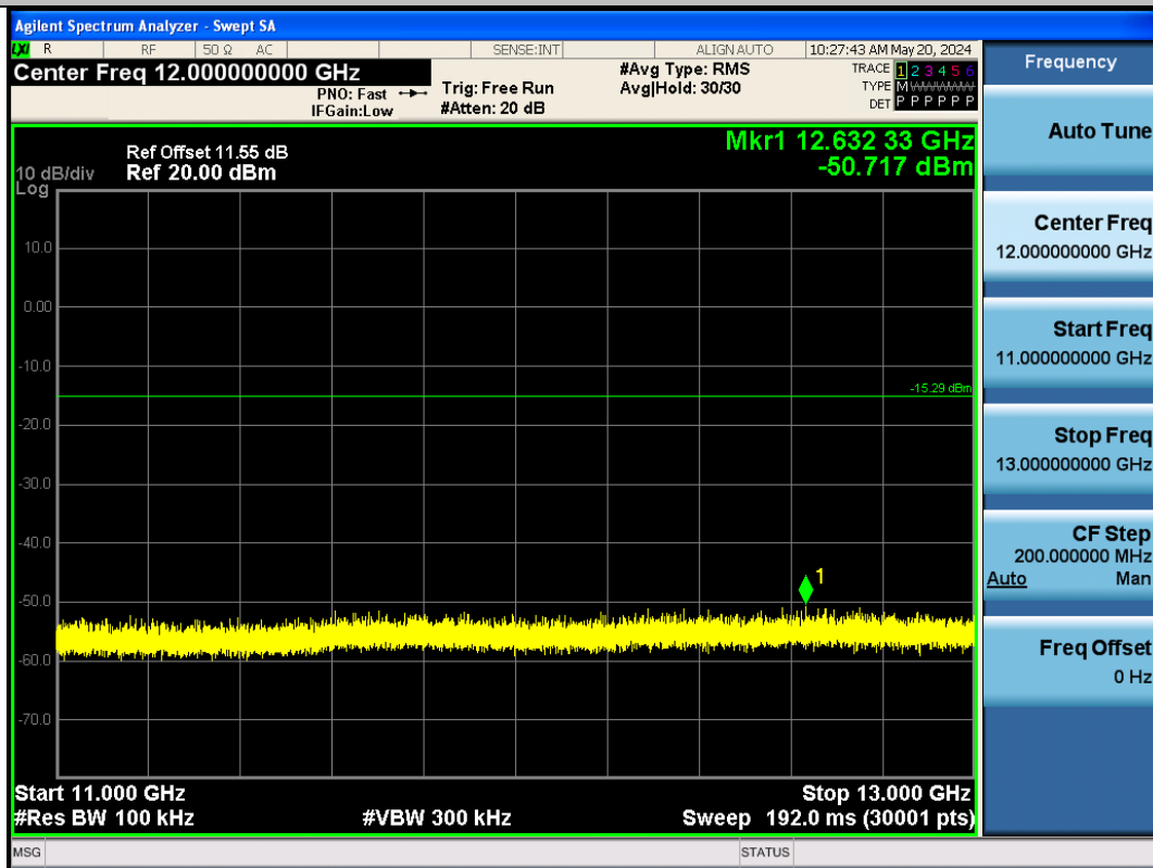
BLE_2M-Ant1-2440-11000~13000-PASS
