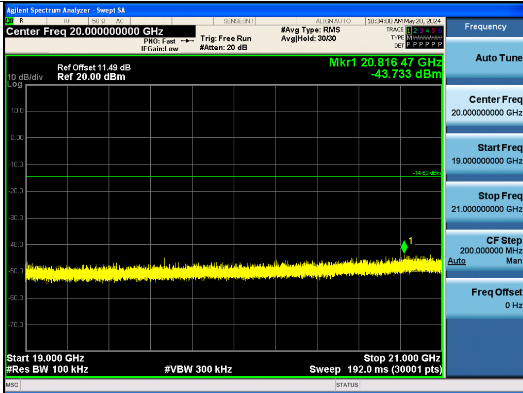
BLE_2M-Ant1-2480-19000~21000-PASS
