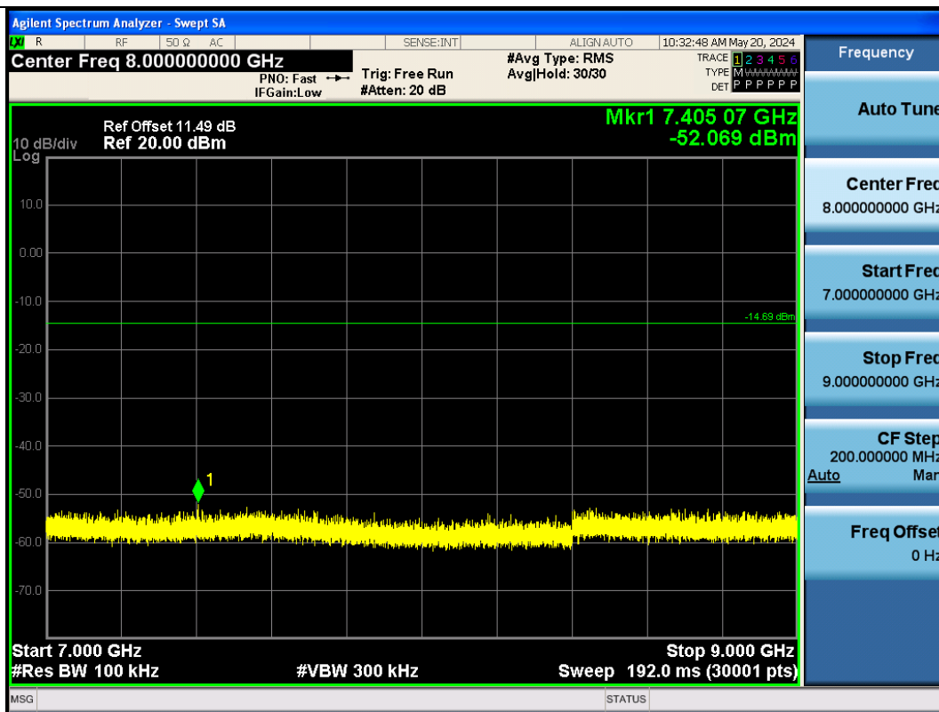
BLE_2M-Ant1-2480-7000~9000-PASS
