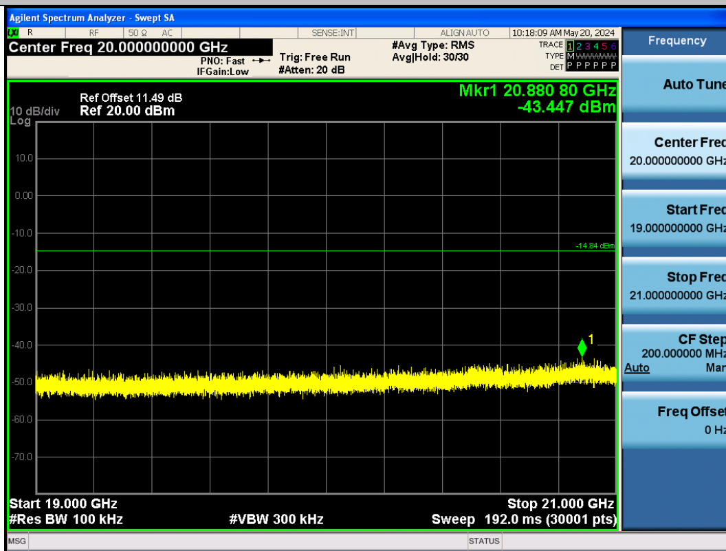
BLE_1M-Ant1-2480-19000~21000-PASS
