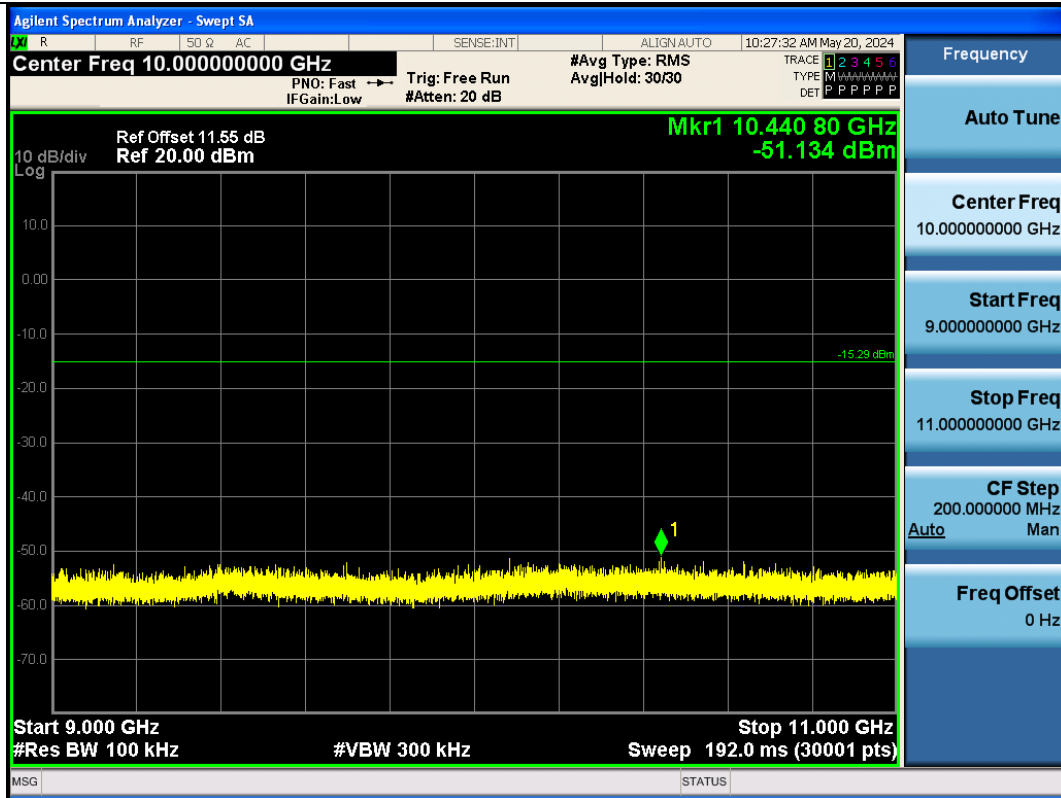
BLE_2M-Ant1-2440-9000~11000-PASS
