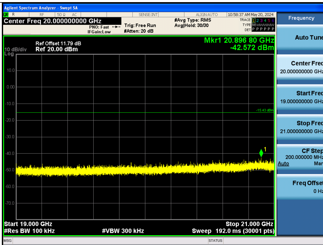
BLE_500K-Ant1-2402-19000~21000-PASS
