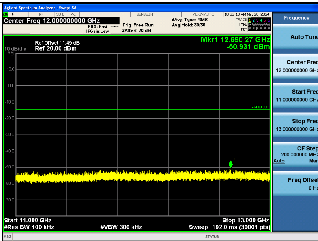
BLE_2M-Ant1-2480-11000~13000-PASS
