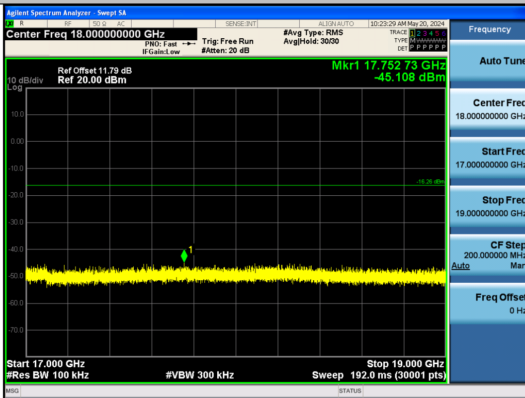
BLE_2M-Ant1-2402-17000~19000-PASS
