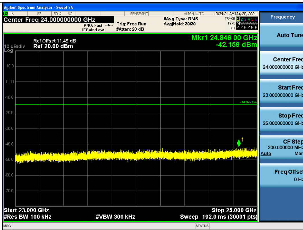
BLE_2M-Ant1-2480-23000~25000-PASS
