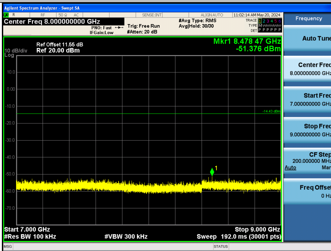
BLE_500K-Ant1-2440-7000~9000-PASS
