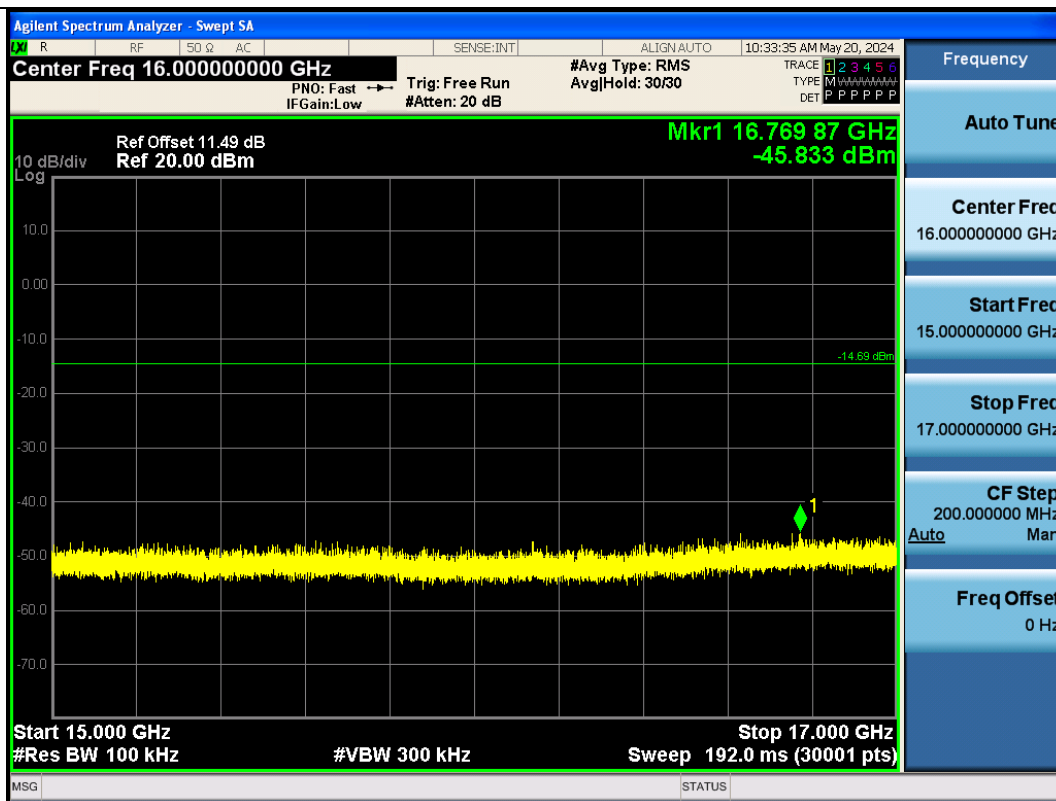
BLE_2M-Ant1-2480-15000~17000-PASS
