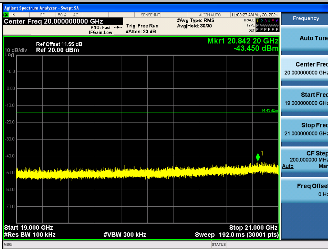
BLE_500K-Ant1-2440-19000~21000-PASS
