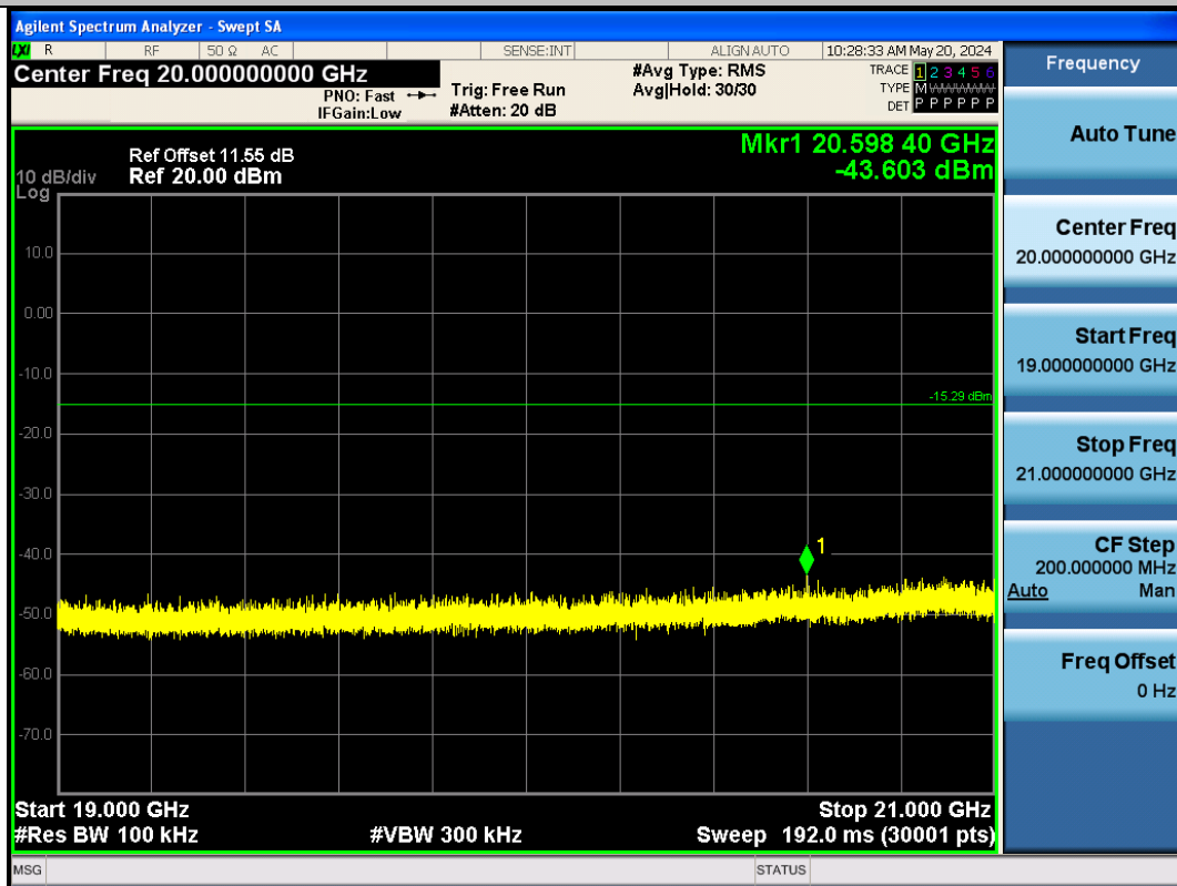
BLE_2M-Ant1-2440-19000~21000-PASS
