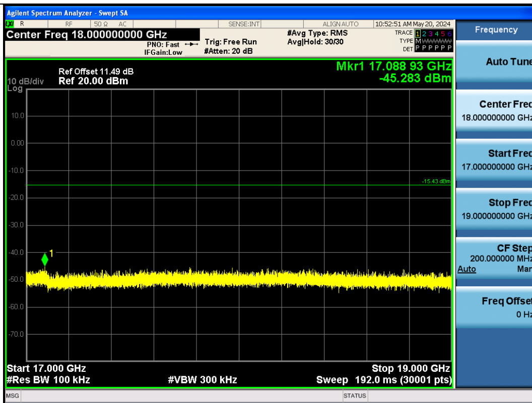
BLE_125K-Ant1-2480-17000~19000-PASS
