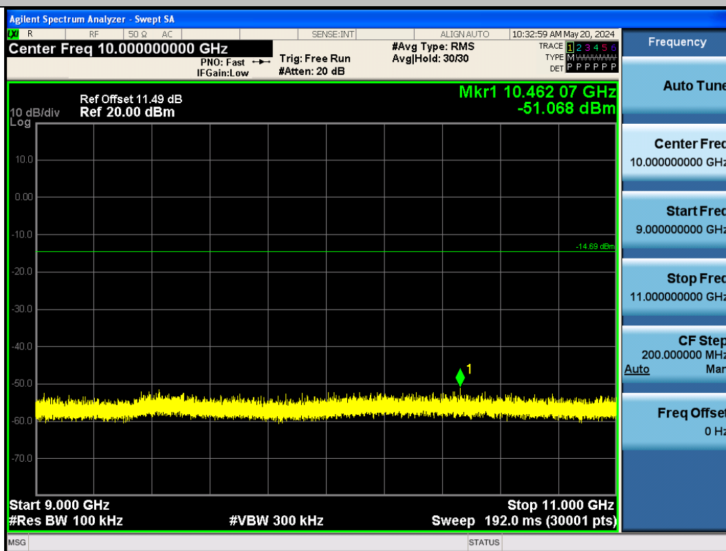
BLE_2M-Ant1-2480-9000~11000-PASS
