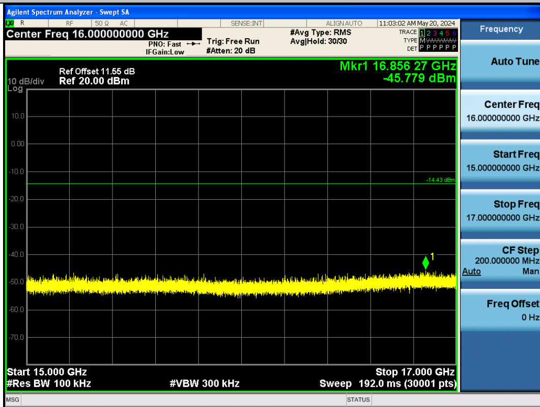
BLE_500K-Ant1-2440-15000~17000-PASS
