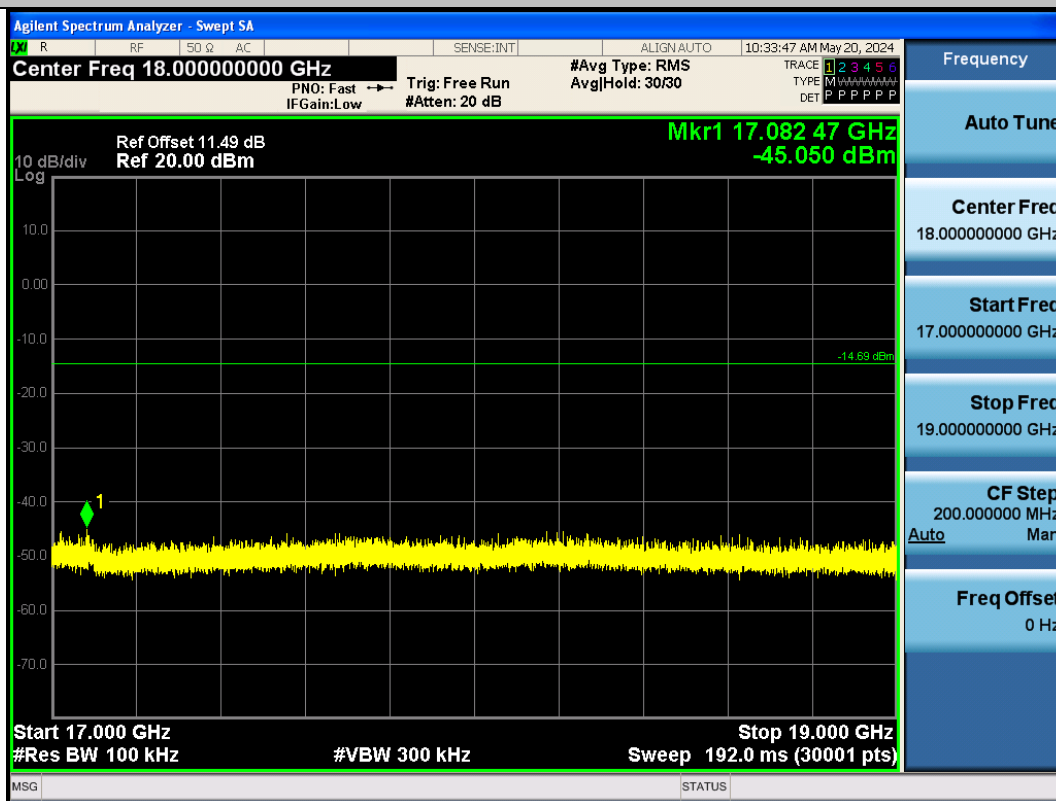
BLE_2M-Ant1-2480-17000~19000-PASS
