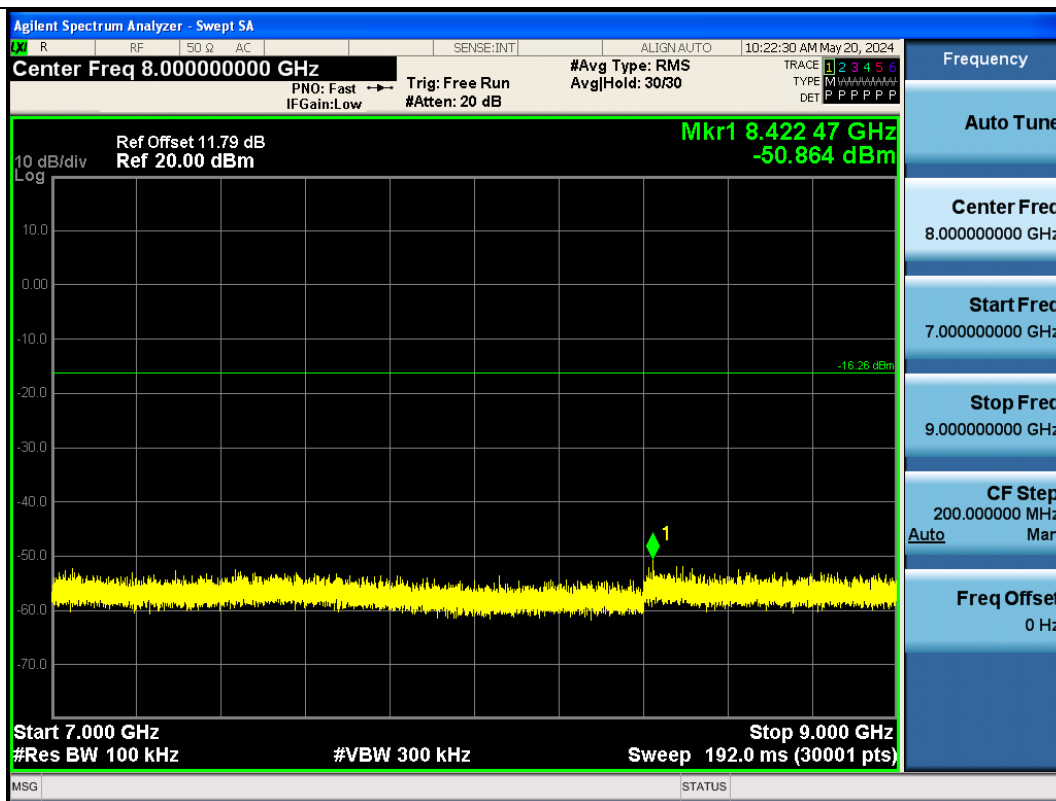
BLE_2M-Ant1-2402-7000~9000-PASS
