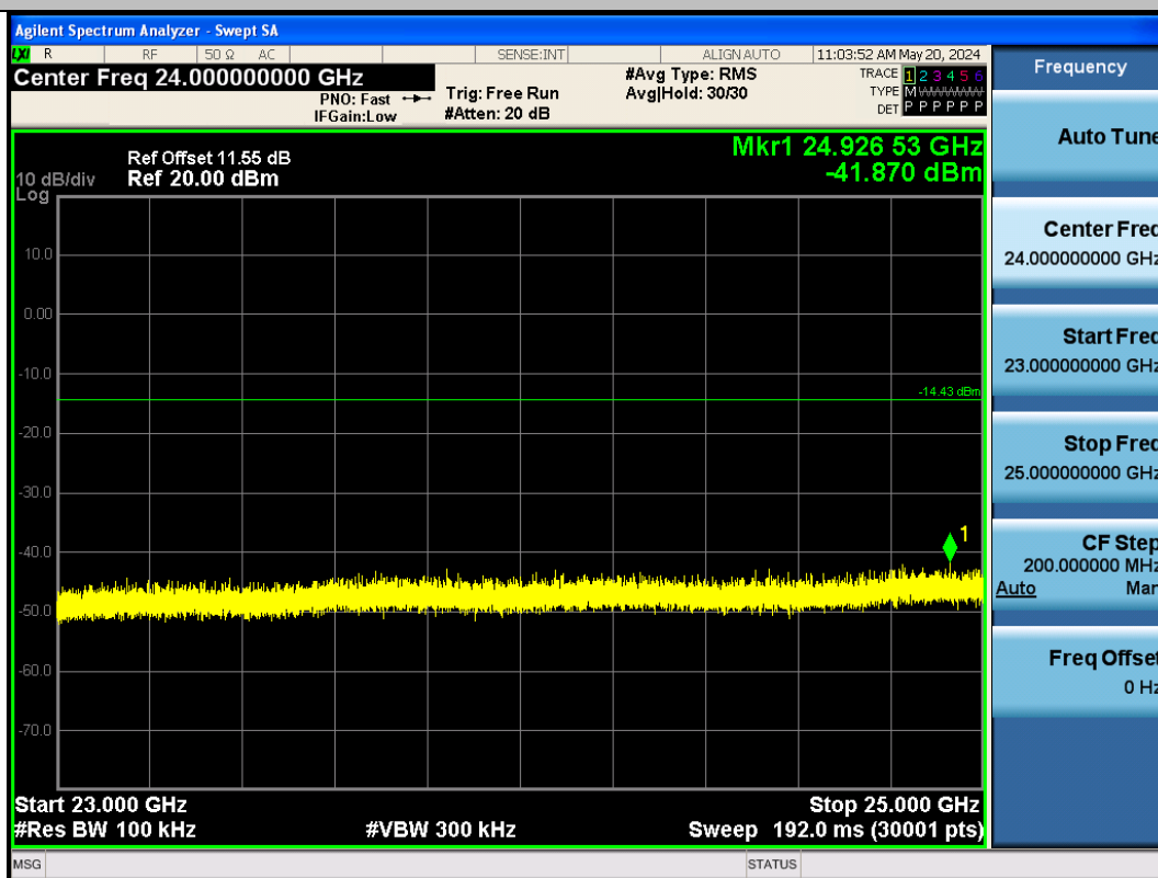
BLE_500K-Ant1-2440-23000~25000-PASS
