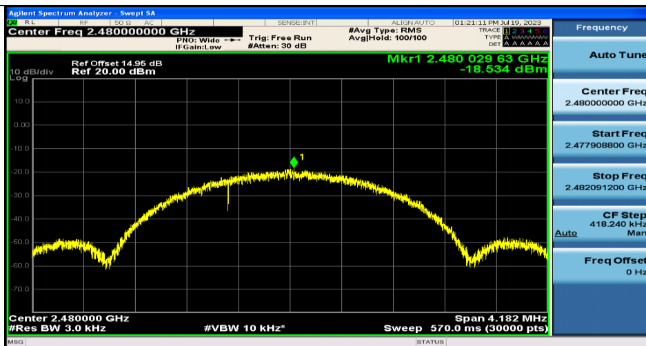
BLE_2M-Ant1-2480
