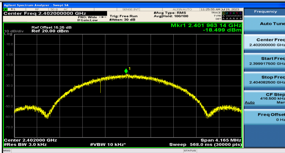
BLE_2M-Ant1-2402
