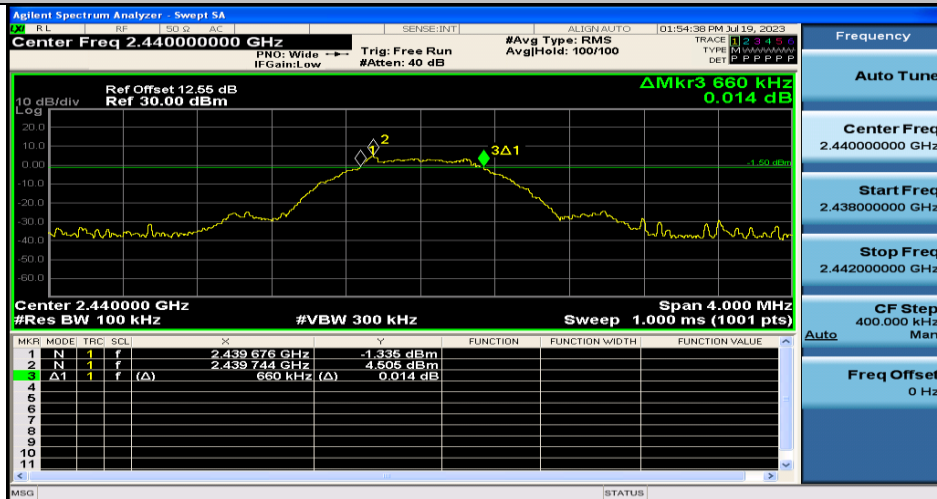
BLE_500K-Ant1-2440
