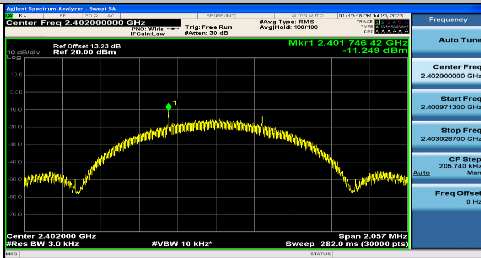
BLE_500K-Ant1-2402
