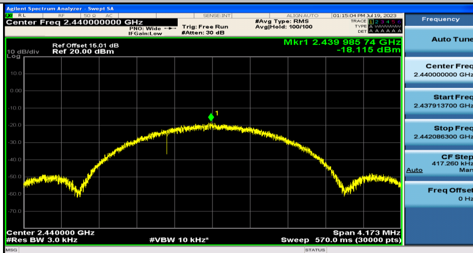
BLE_2M-Ant1-2440
