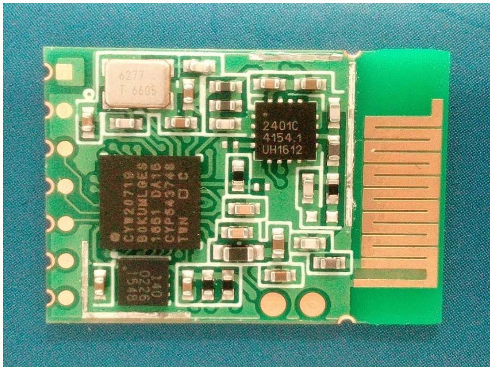
(2) EUT Photo (CYBLE-413136-01)
