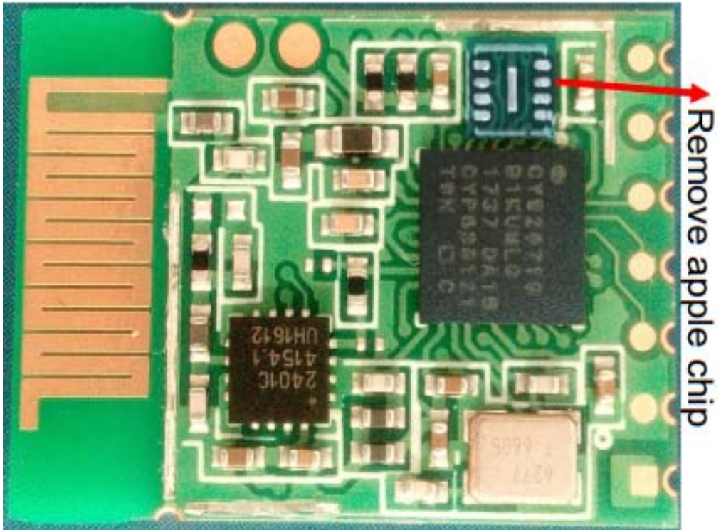
(5) EUT Photo (CYBLE-473148-01)
