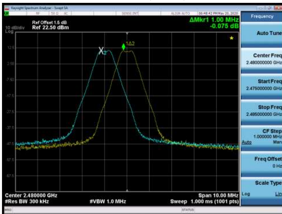
Mode 1 CH78(2480MHz)
