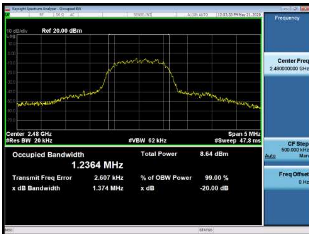
Mode 3 CH78(2480MHz)
