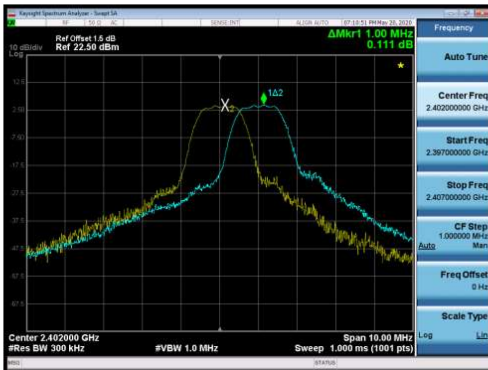
Mode 2 CH00(2402MHz)
