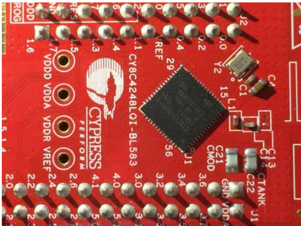
(2) EUT Photo CY8CKIT-143A
