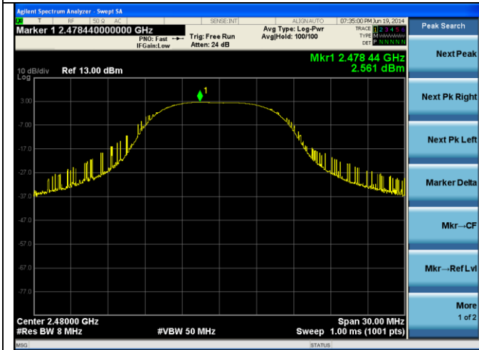
PWR-Zigbee 2480
