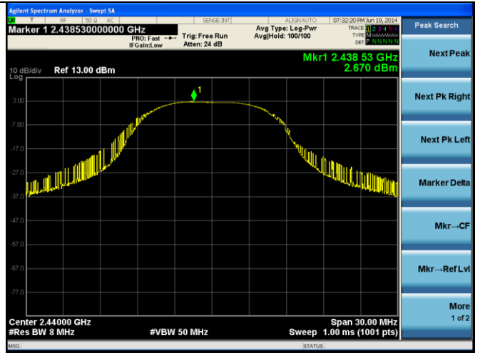
PWR TX-Zigbee 2440
