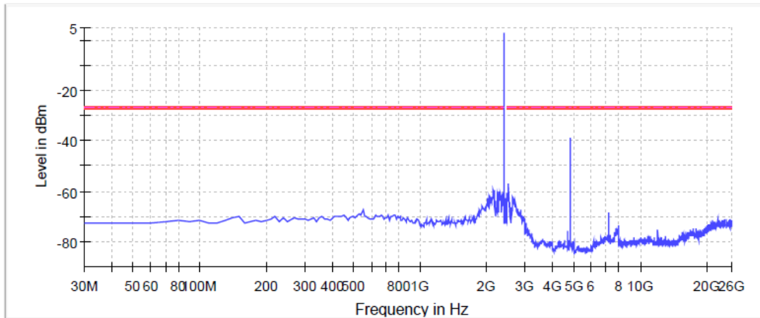
BT LE 1 Mbps Ch 00
