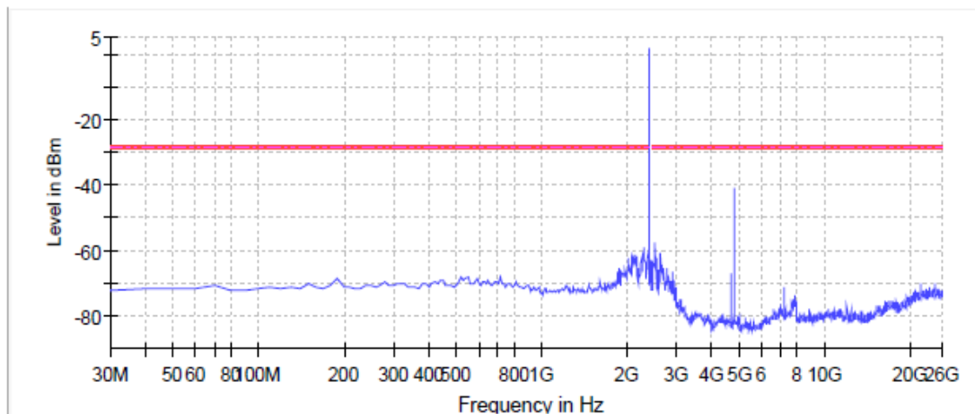
BT LE 2 Mbps Ch 00
