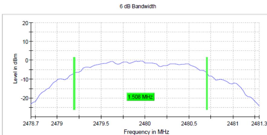
BT LE 2 Mbps Ch 39
