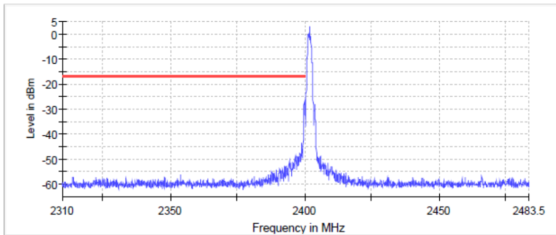
BT LE 2 Mbps Ch 00 Band Edge
