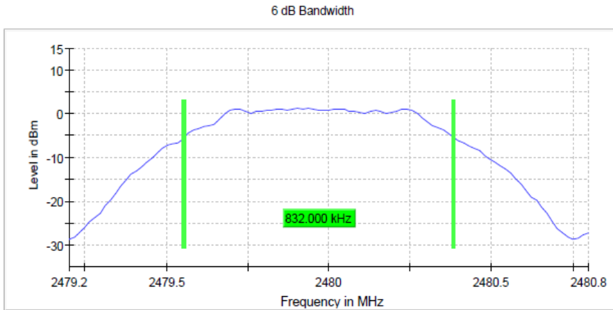
BT LE 1 Mbps Ch 39
