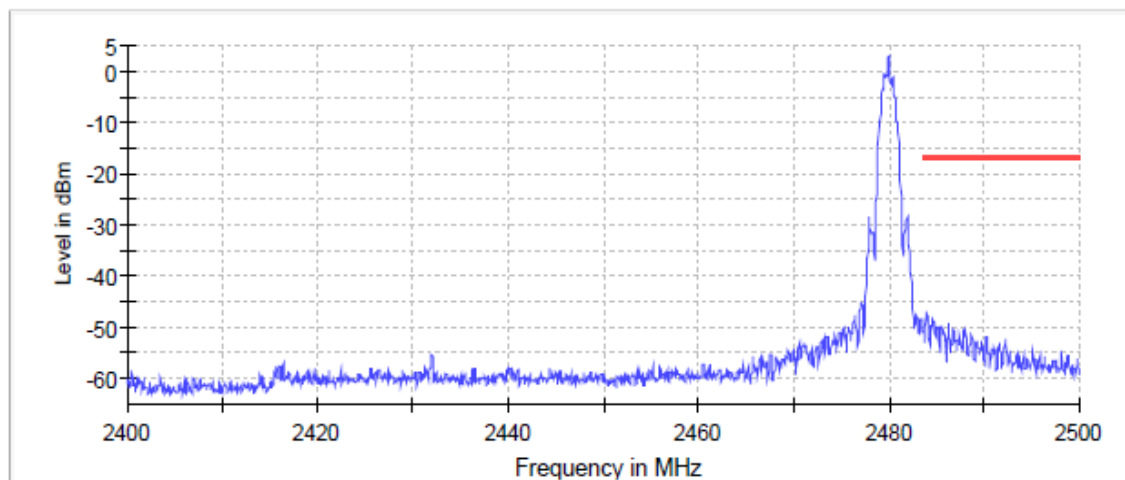
BT LE 2 Mbps Ch 39 Band Edge
