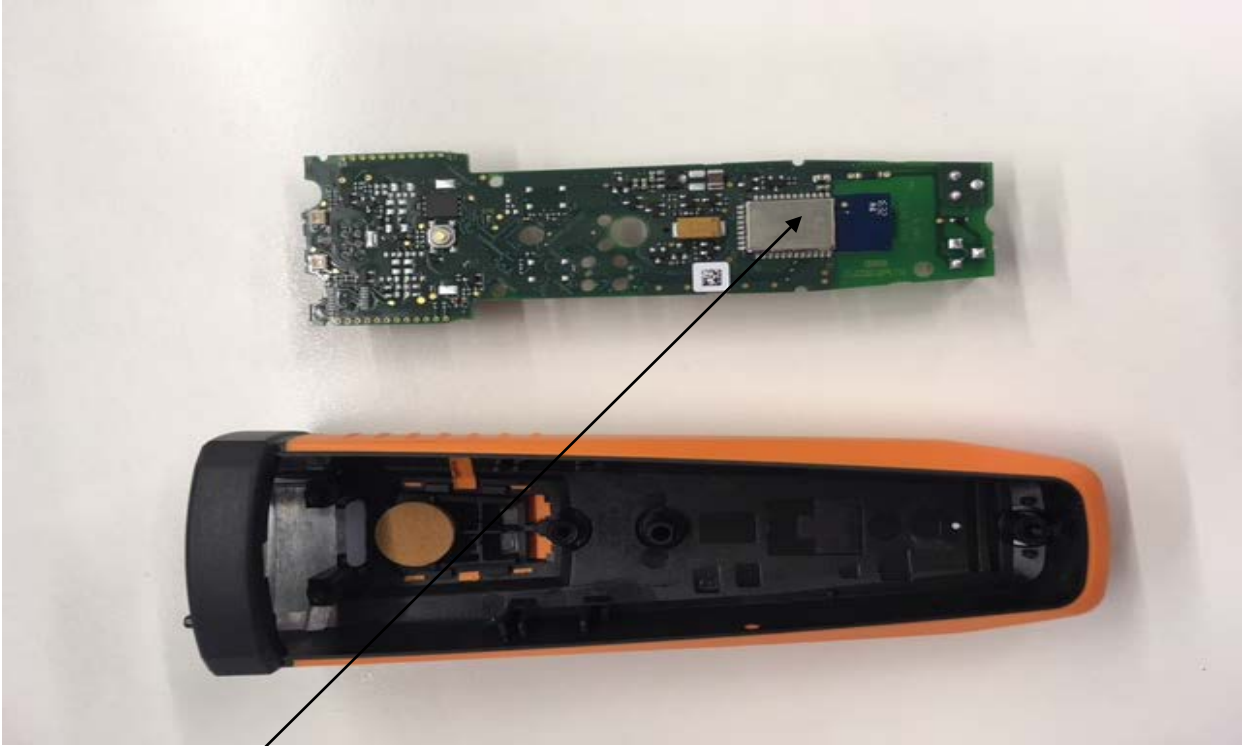
Module + Antenna
