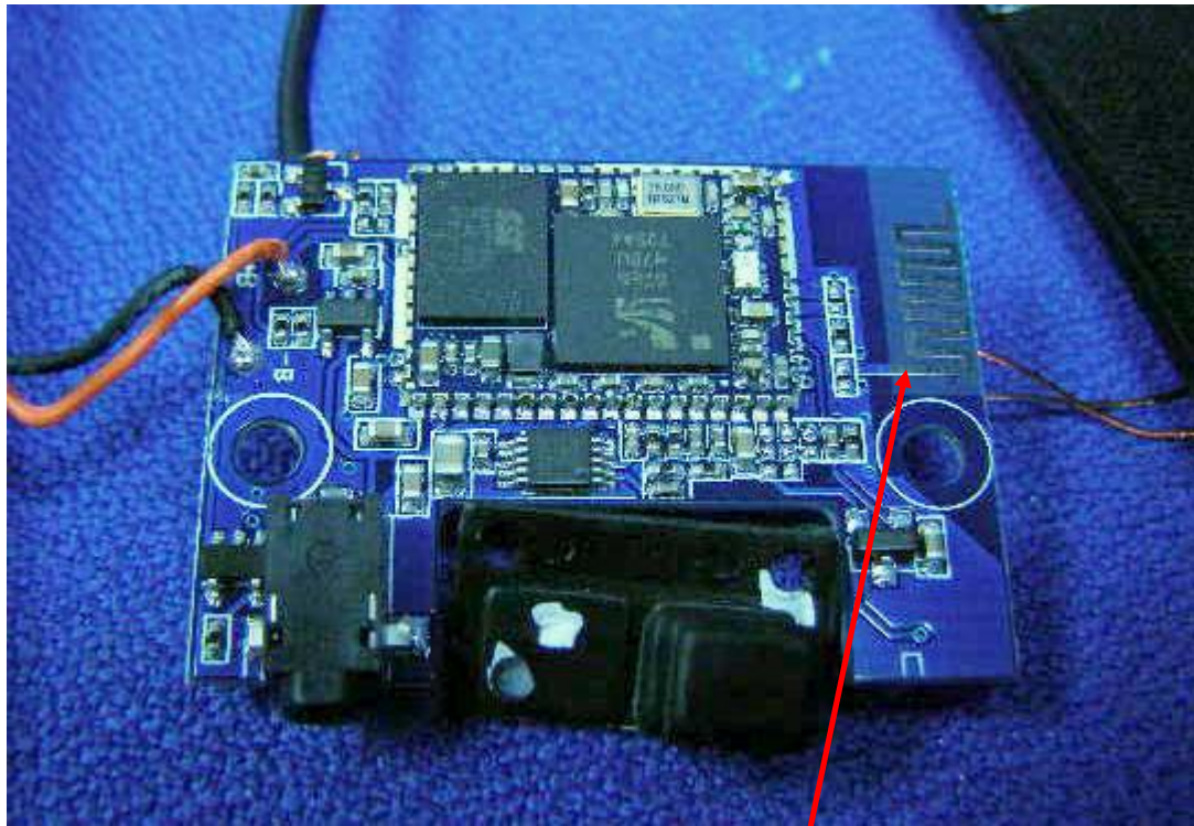
Antenna
