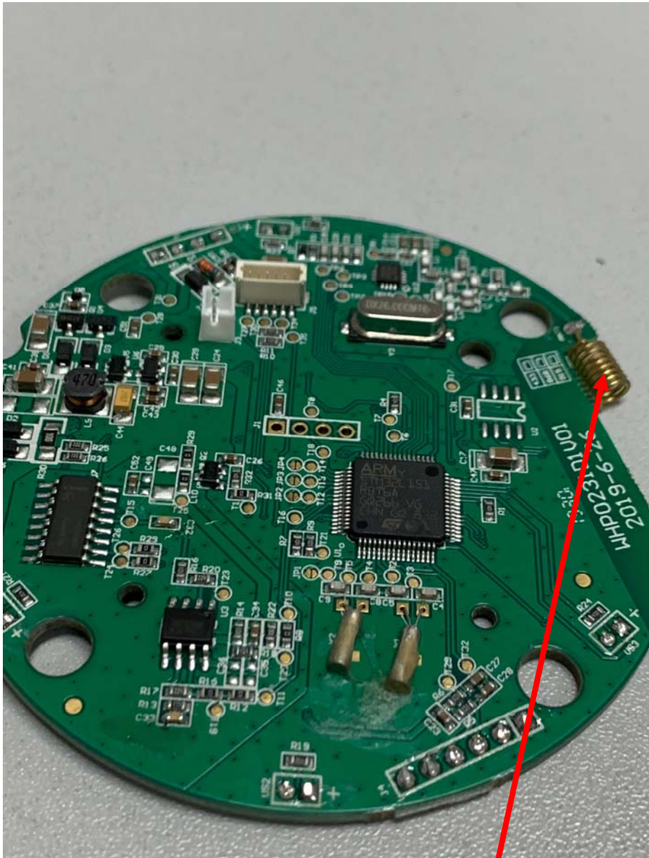
Antenna
