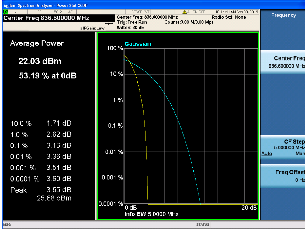
WCDMA850 & Channel: 4183
