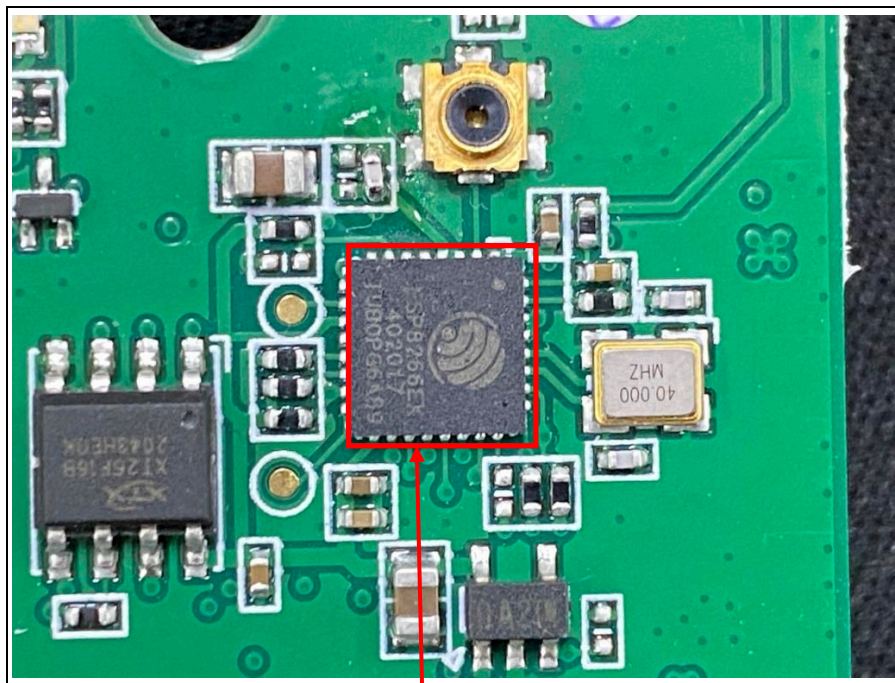
WLAN Module
