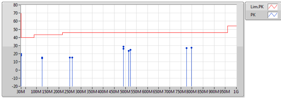
RE TX below 1GHz;Band:5.2G;VHT80;BWch:80MHz;Nss:1.(M0);Nant:2;Ch:5210MHz;AC Adapter 1
