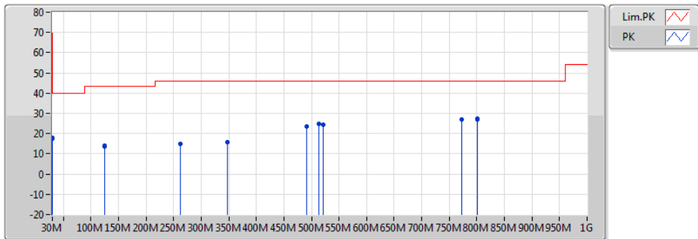
RE TX below 1GHz;Band:5.2G;VHT80;BWch:80MHz;Nss:1.(M0);Nant:2;Ch:5210MHz;AC Adapter 2
