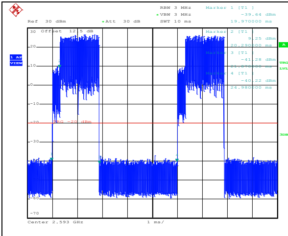
PUSC, QPSK 3/4, BW 5MHz
