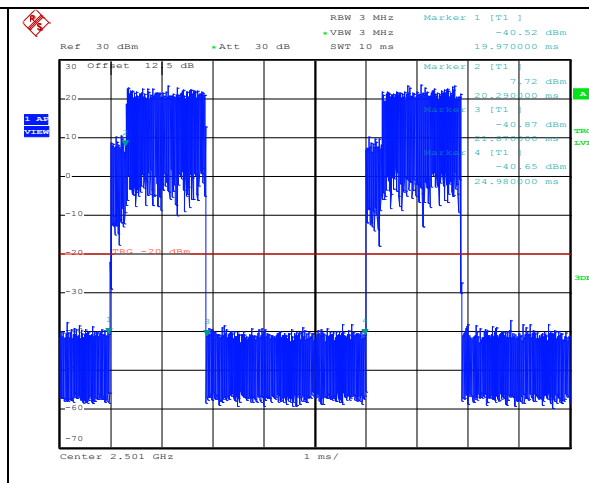
PUSC, 16QAM 1/2, BW 10MHz
