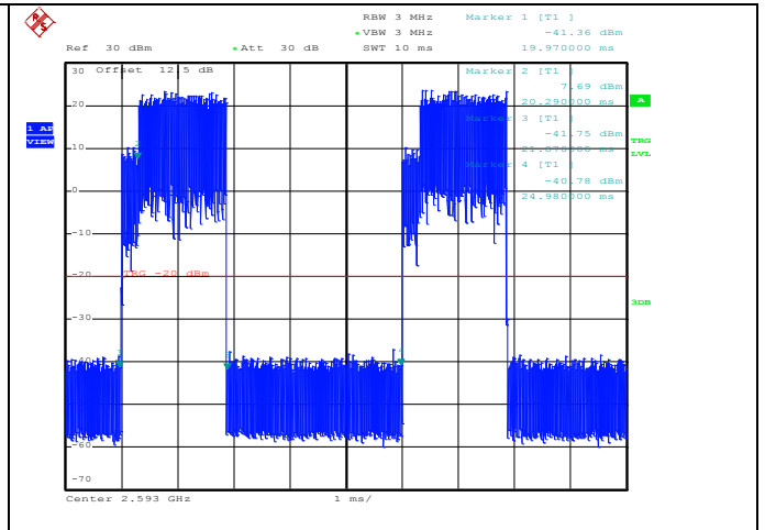
PUSC, 16QAM 3/4, BW 10MHz
