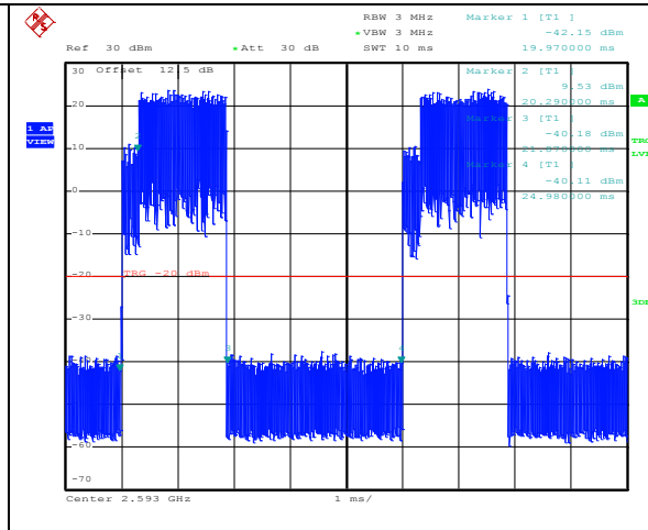
PUSC, QPSK 3/4, BW 10MHz
