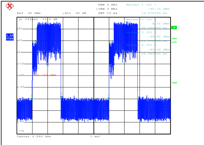
PUSC, 16QAM 3/4, BW 5MHz
