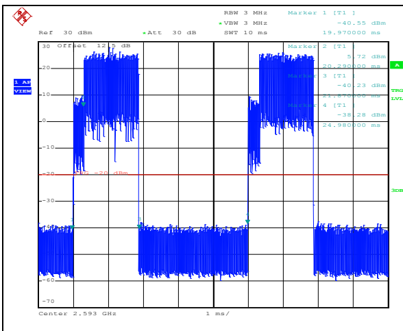
PUSC, 16QAM 1/2, BW 5MHz
