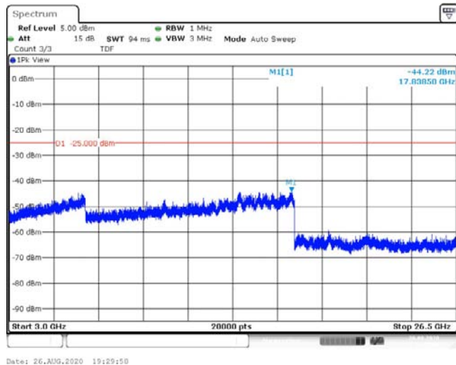
Band41-20MHz-QPSK-41490-1RB#0-Range3:3000~26500MHz--44.22-PASS
