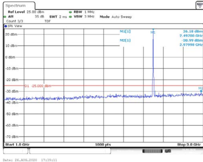
Band41-5MHz-QPSK-39675-1RB#0-Range2:1000~3000MHz--30.99-PASS
