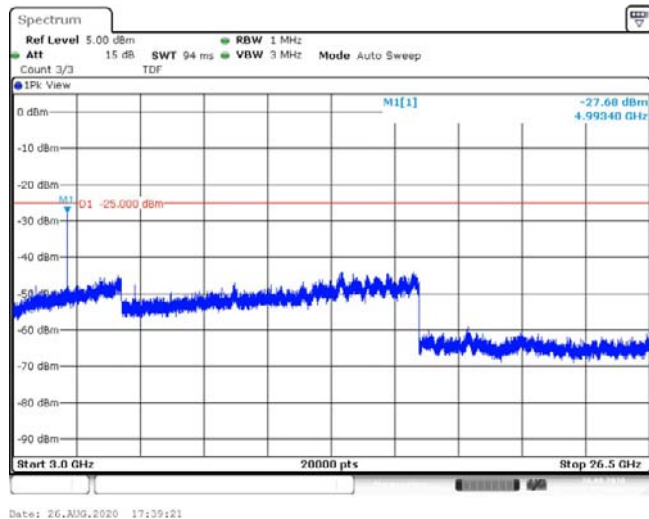
Band41-5MHz-QPSK-39675-1RB#0-Range3:3000~26500MHz--27.68-PASS
