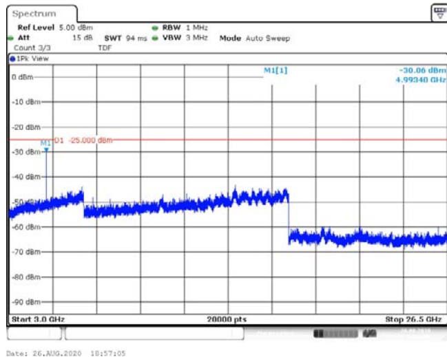
Band41-10MHz-QPSK-39700-1RB#0-Range3:3000~26500MHz--30.06-PASS
