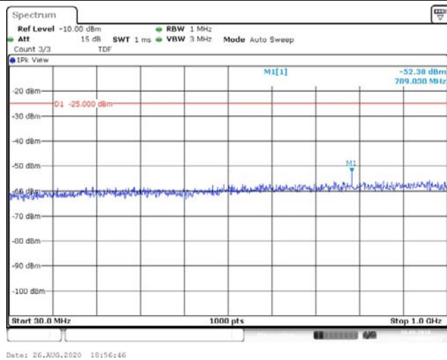
Band41-10MHz-QPSK-39700-1RB#0-Range1:30~1000MHz--52.38-PASS
