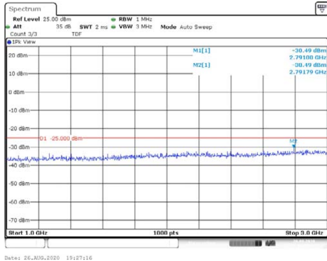
Band41-20MHz-QPSK-39750-1RB#0-Range2:1000~3000MHz--30.49-PASS
