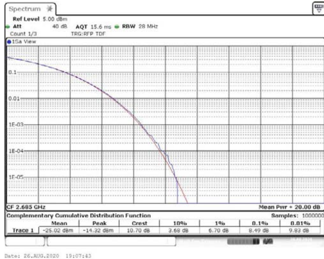
Band41-10MHz-QPSK-41540-50RB#0-8.49-13-PASS
