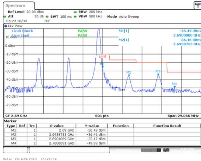
Band41-10MHz-QPSK-41540-1RB#49--26.49,-36.46,-35.17,-49.99-PASS
