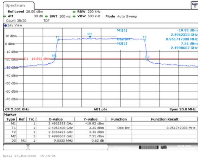
Band41-10MHz-QPSK-39700-50RB#0-8.952-9.533-PASS
