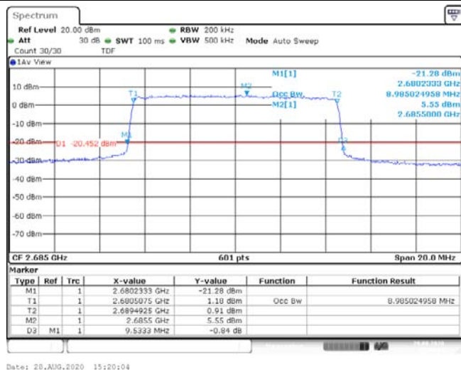
Band41-10MHz-QPSK-41540-50RB#0-8.985-9.533-PASS
