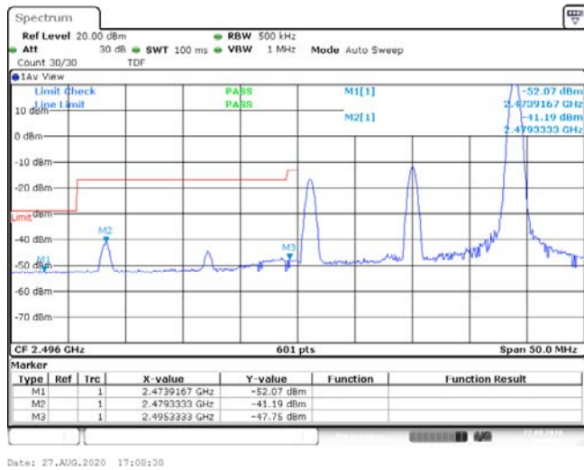
Band41-20MHz-QPSK-39750-1RB#99--52.07,-41.19,-47.75-PASS
