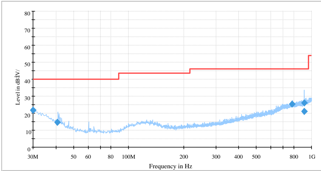
Auto Test (FCC 15.109)
