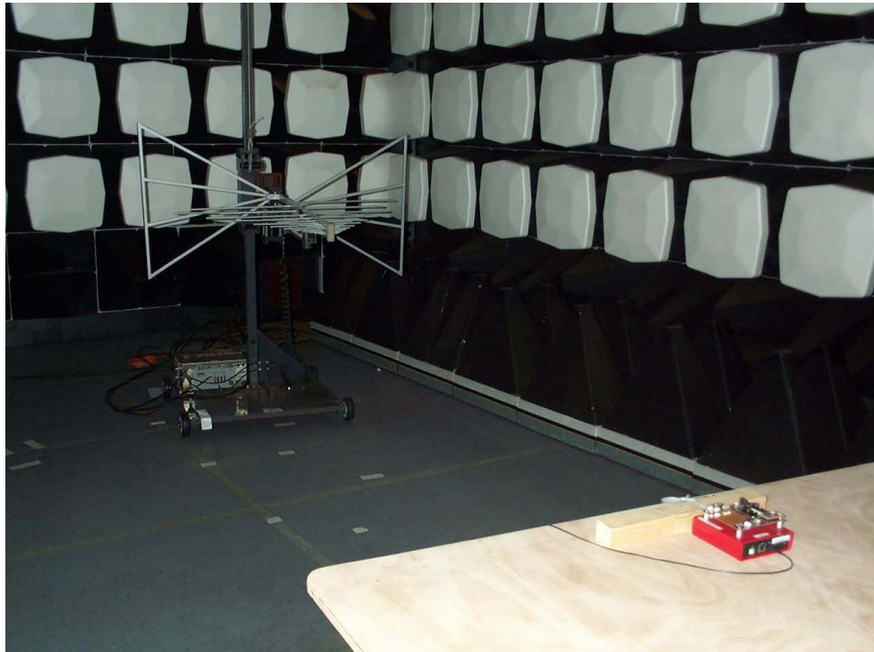
Bild 1. El. Funkstörfeldstärke [emission, radiated disturbance]
