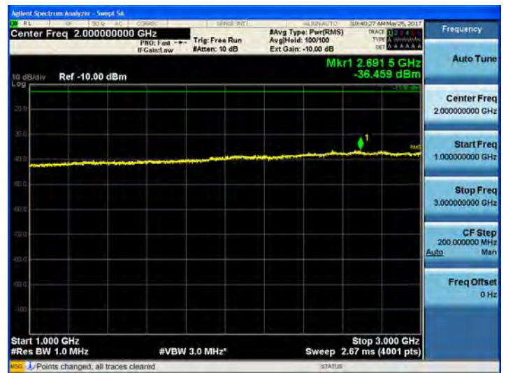
1 GHz ~ 3 GHz
