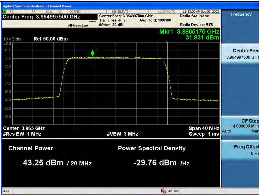
PSD / C-Band(Ant1) / Downlink / 5G NR 20 MHz
