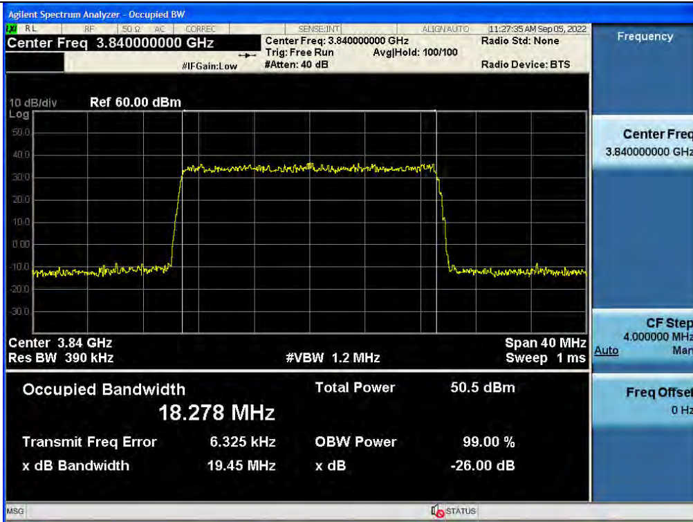
Output / C-Band(Ant1) / Downlink / 5G NR 20 MHz
