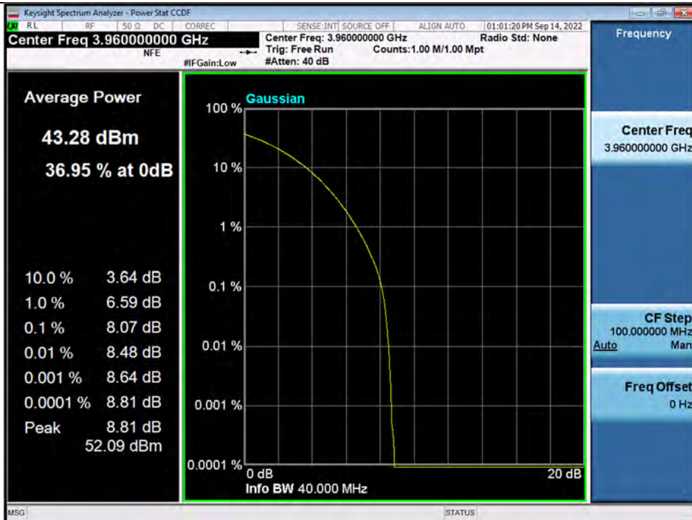
PAPR / C-Band(Ant1) / Downlink / 5G NR 40 MHz
