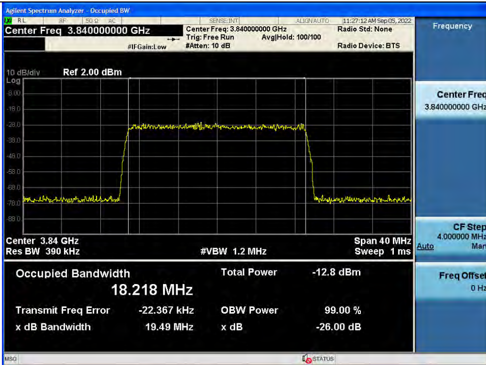
Input / C-Band(Ant1) / Downlink / 5G NR 20 MHz
