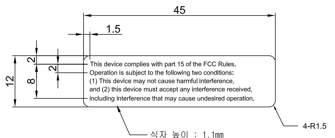
[ HRDU용 FCC 선언 문구 Label ]
