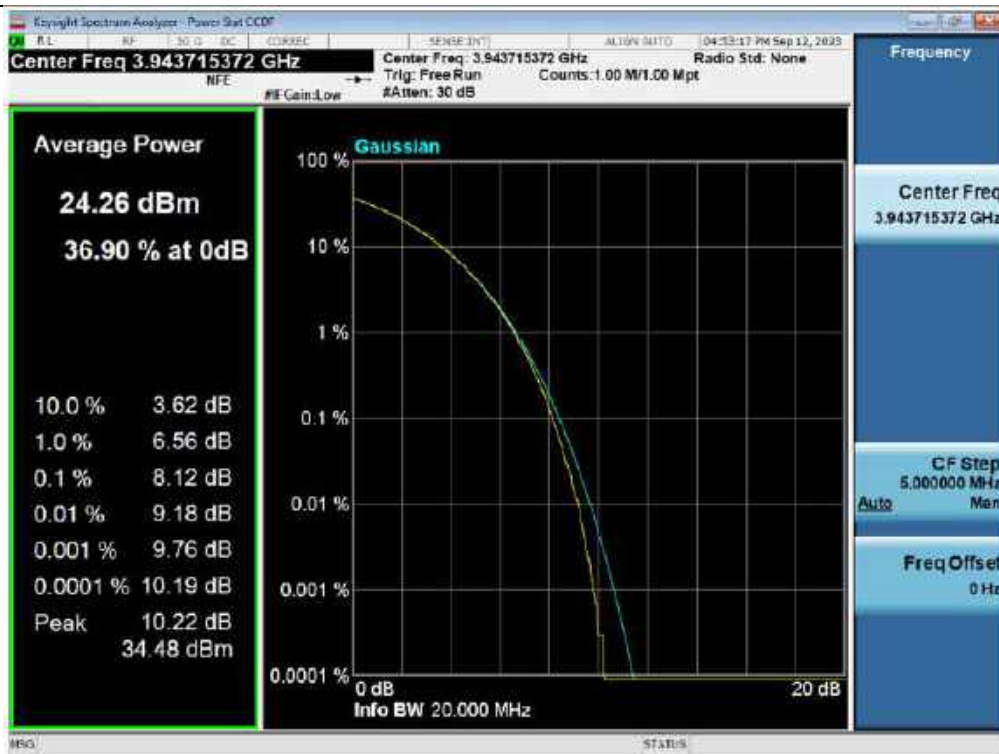
PAPR / 3.7 GHz Service (ANT 1) / Downlink / 5G NR 20 MHz
