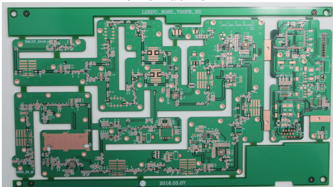
UL PCB Bare - TOP
