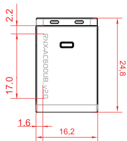
尺寸图
