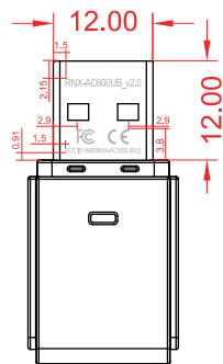
结构图
