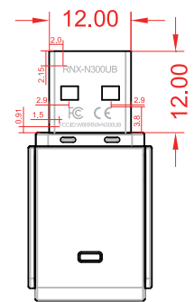
结构图
