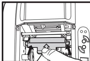
将集尘胶卷器放於机台内进行清洁 (请至驱动程式中执行)
