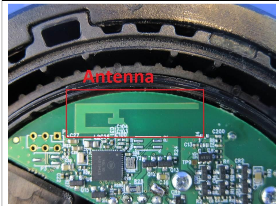
Antenna
