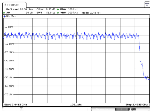
2442-2480 MHz
