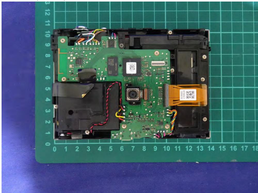
(12) EUT Photo(Print:TP)
