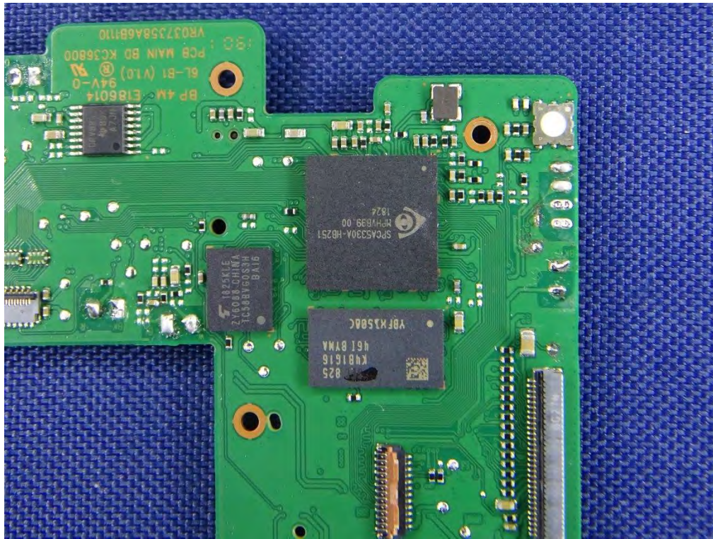
(18) EUT Photo
