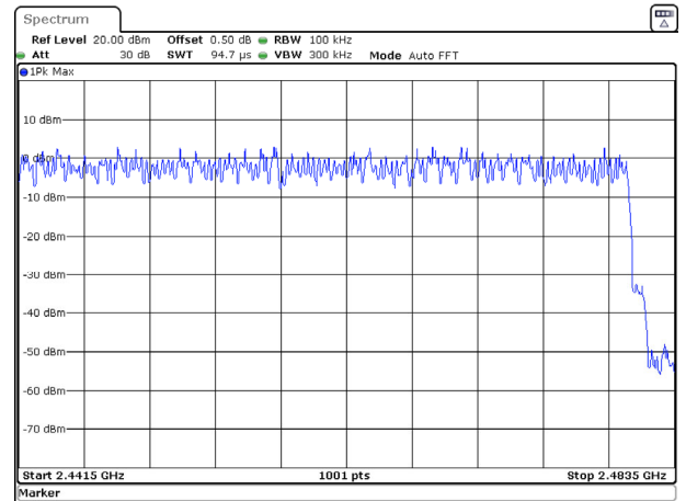
2480 MHz
