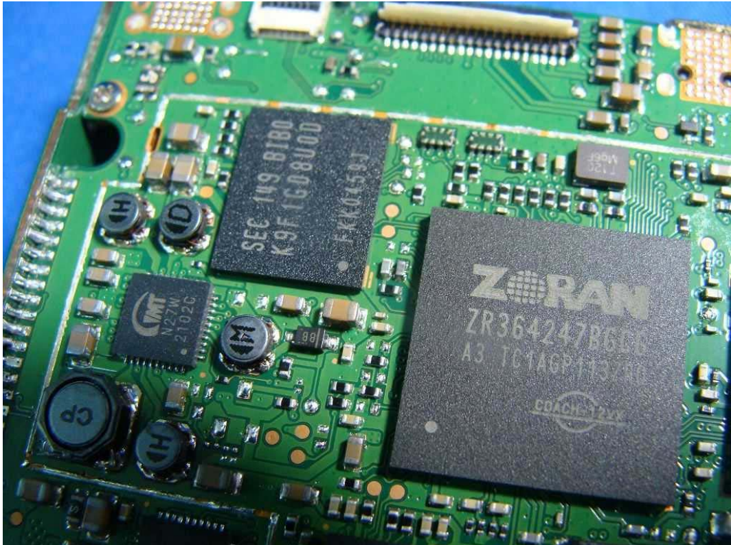
(19) EUT Photo
