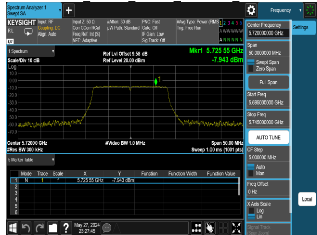
802.11a 20MHz Chain1 5720MHz UNII 3
