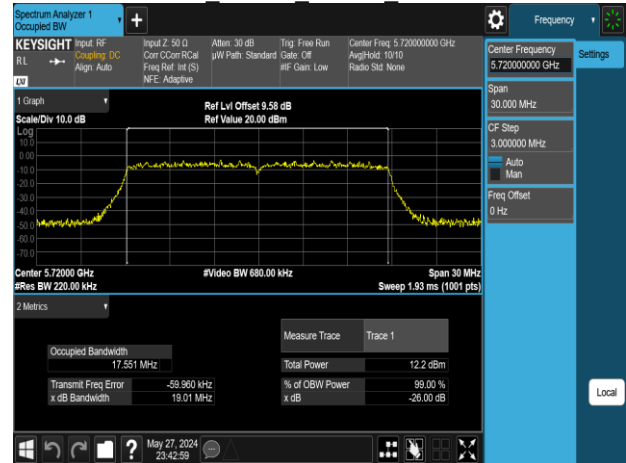
802.11n 20MHz Chain1 5720MHz
