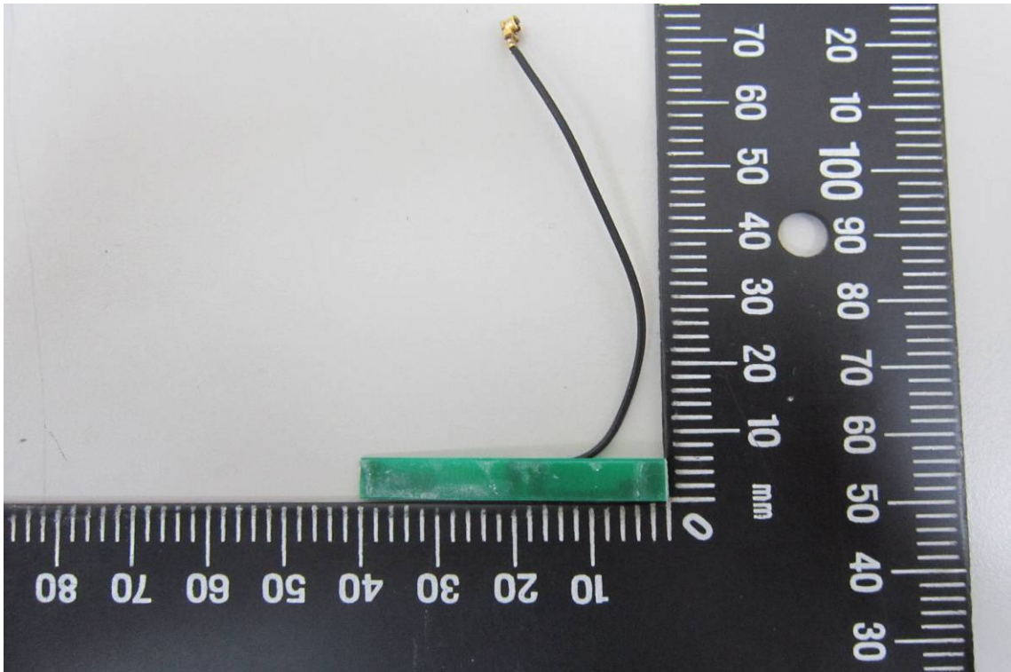
WLAN Antenna-Aux-3
