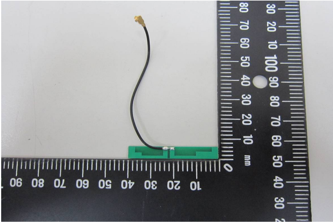
WLAN Antenna-Aux-3
