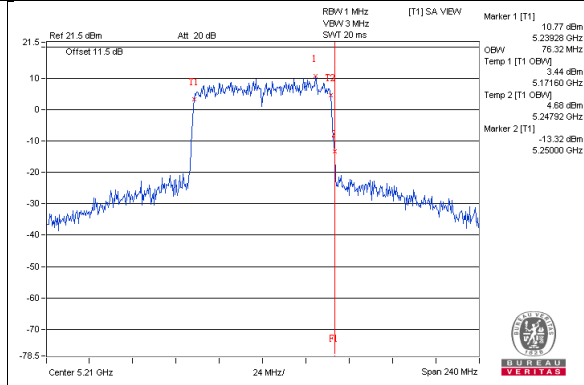
802.11ac(VHT80+80) / Chain 1 : CH42
