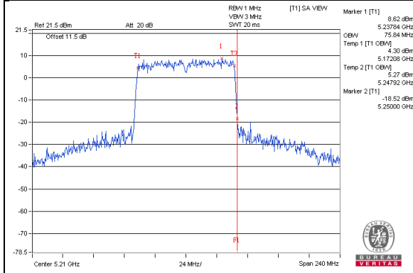
802.11ac(VHT80+80) / Chain 0 : CH42
