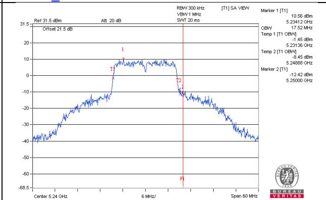
802.11ac(VHT20)_Chain1 / CH48
