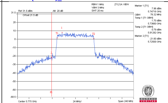
802.11ac(VHT80)_Chain1 / CH155
