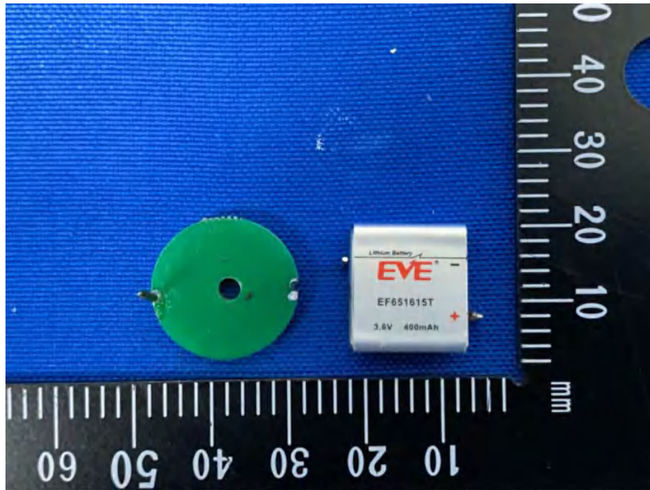
(9) EUT Photo
